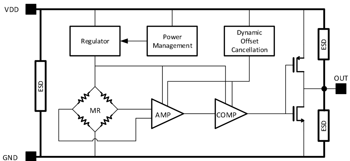
图 2 模块/线路图
