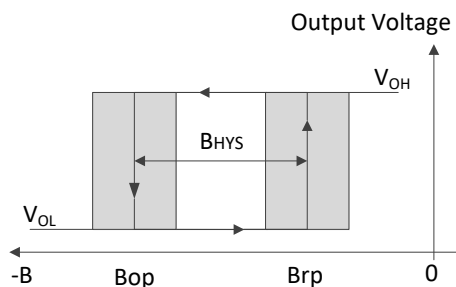
S0T23-3L 输出状态
