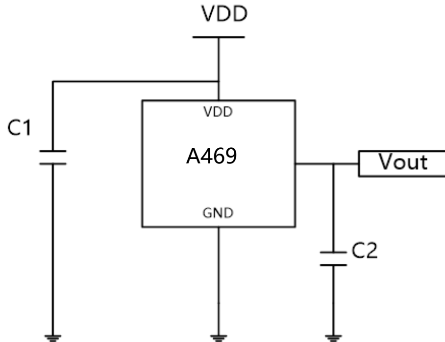
典型应用电路
