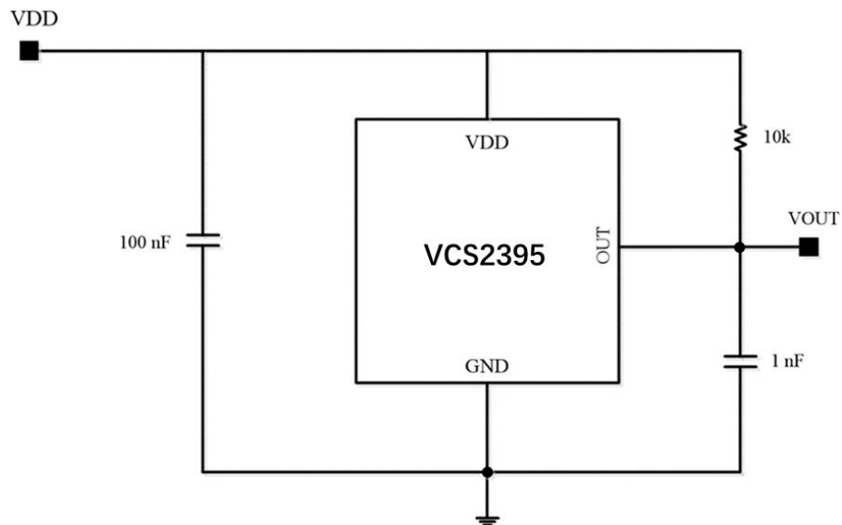
图 4 典型应用图
