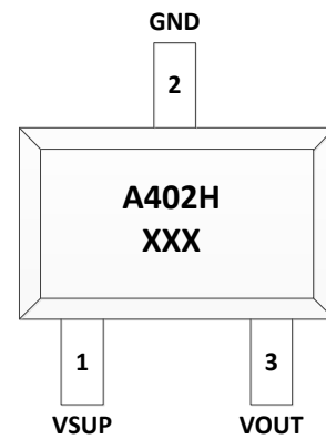
SOT23-3L
