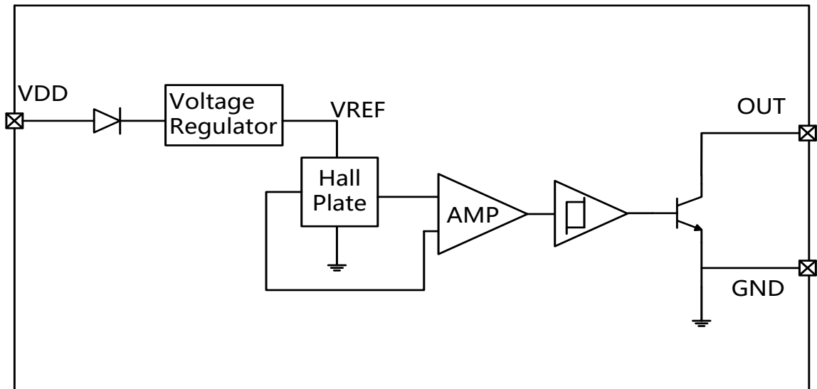
AR402H功能框图
