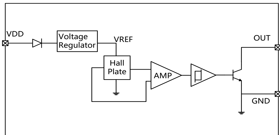
AR422 功能框图
