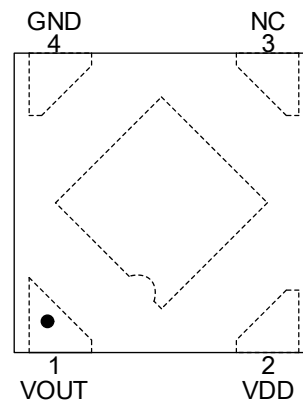
DFN4L 封装
