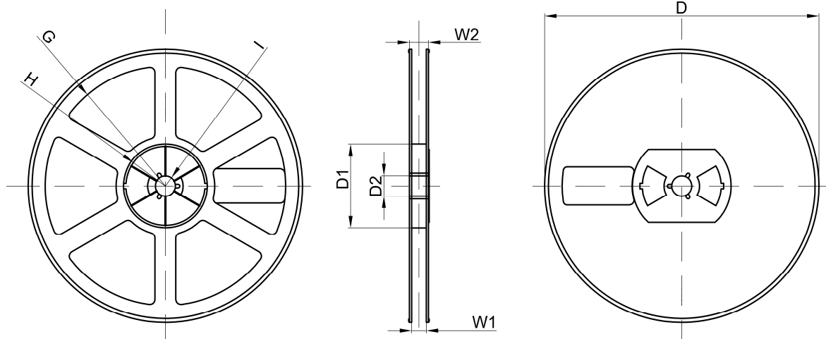
SOT23-3 卷盘
