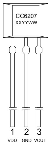
TO-92S 封装
