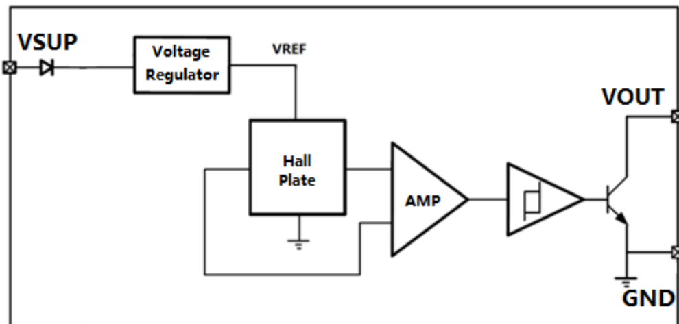
AR41F 功能框图
