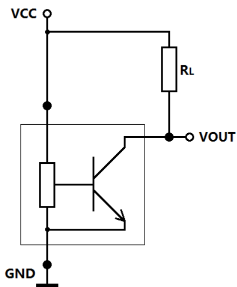
应用电路 1
