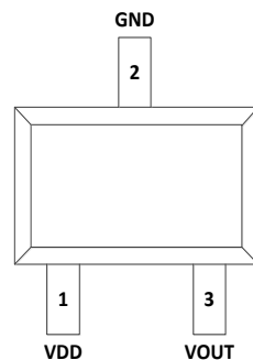
SOT23
