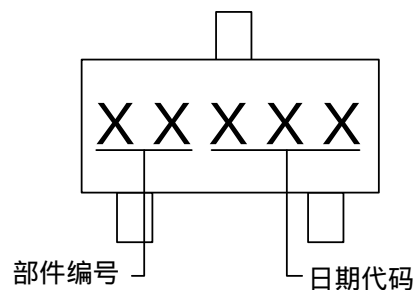
2) SOT-23
