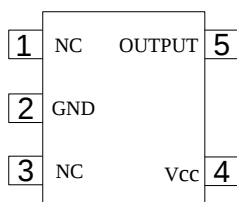
SOT553
