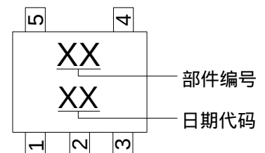
3) SOT553
