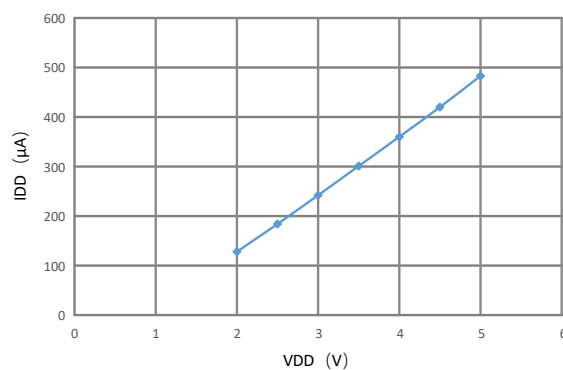
静态电流 vs. 工作电压
