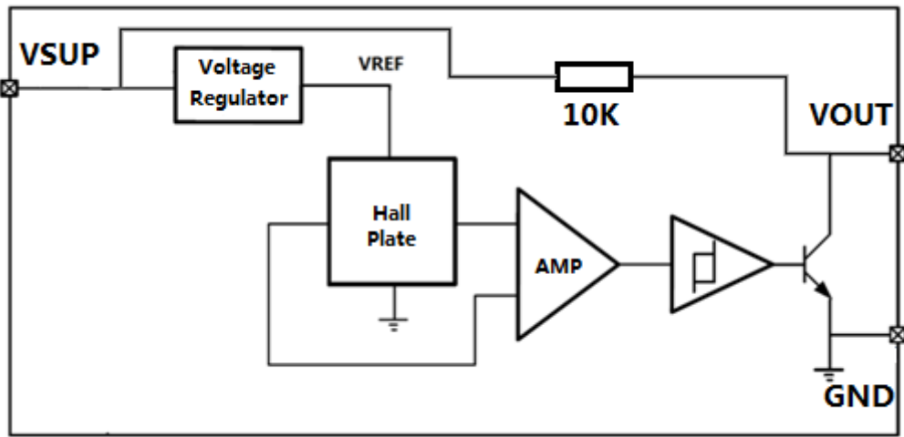
AR402F功能框图
