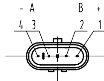
编码器
