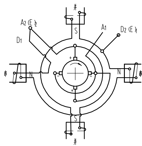
电机接线原理图 换向器端视
