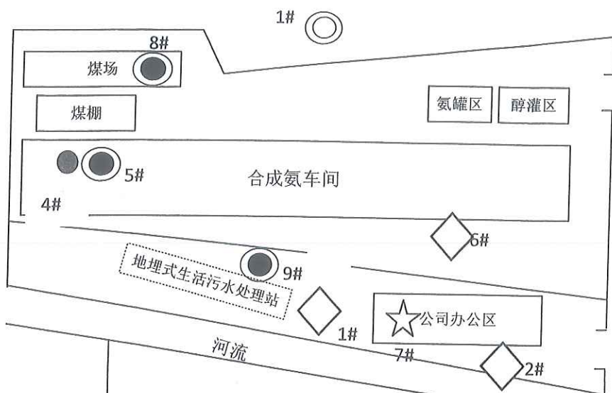
2021. 4. 6-8 威海恒邦化工有限公司现场采样简图
