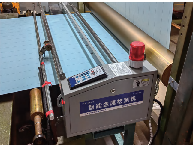
无传动式检针机 No transmission type
