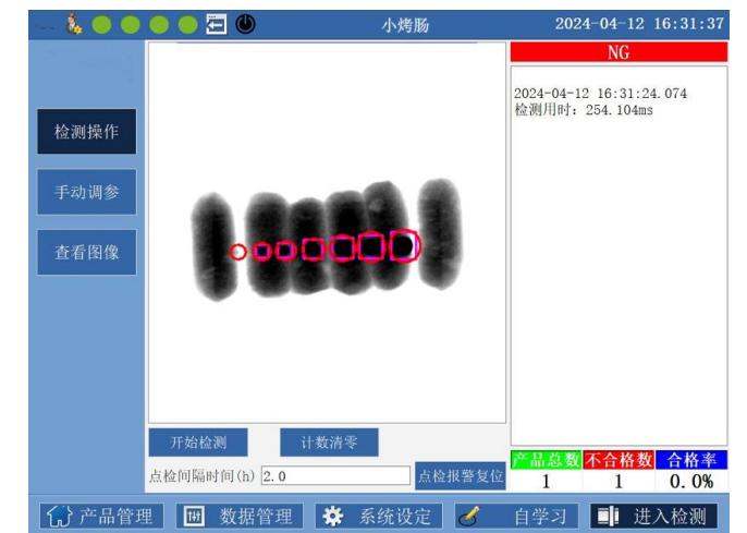
软件检测界面 Detecting image interface
