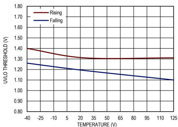
图 10 UVLO 阈值
