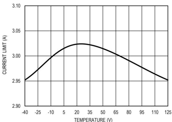
图 12 输出限流值和温度的关系
