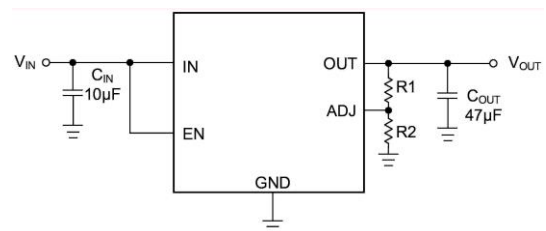
图 2 典型应用
