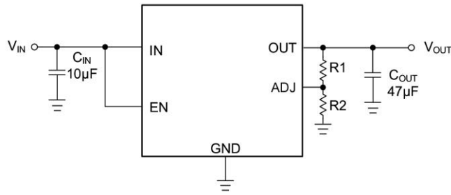
图 16 由外部电阻决定的输出电压
