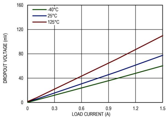
图 6 压差电压和负载的关系, V_{OUT} = 1.5V
