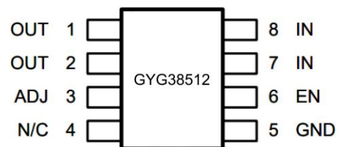
图1 eSOP8/CQF8引脚图
