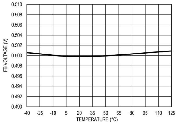
图 4 FB 引脚电压和温度的关系
