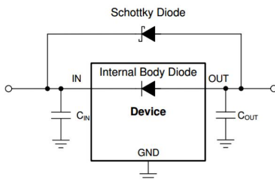
图 18 反向电流保护应用电路
