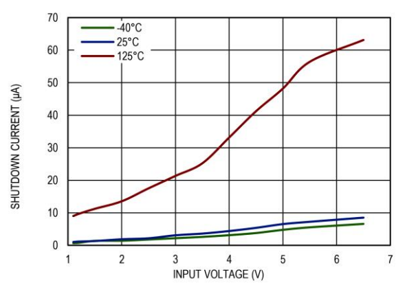
图 9 停机静态电流和输入电压的关系
