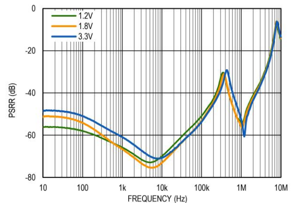
图 13 PSRR, V_{IN} = V_{OUT} + 0.4V , I_O = 1.5A
