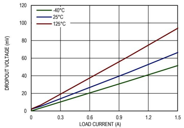
图 7 压差电压和负载的关系, V_{OUT} = 5.0V
