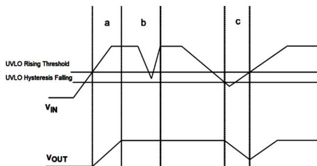
图 17 欠压锁定条件和输出变化
