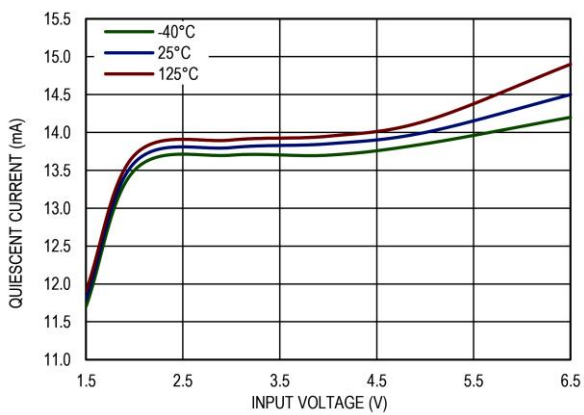
图 8 静态电流和输入电压的关系, I_{OUT} = 1mA
