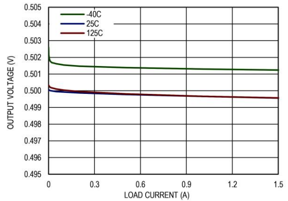
图 5 负载调整率
