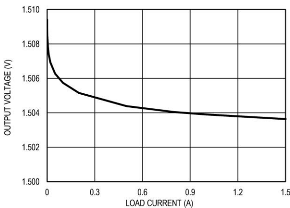
图 9 1.5V 输出电压 VS 负载电流
