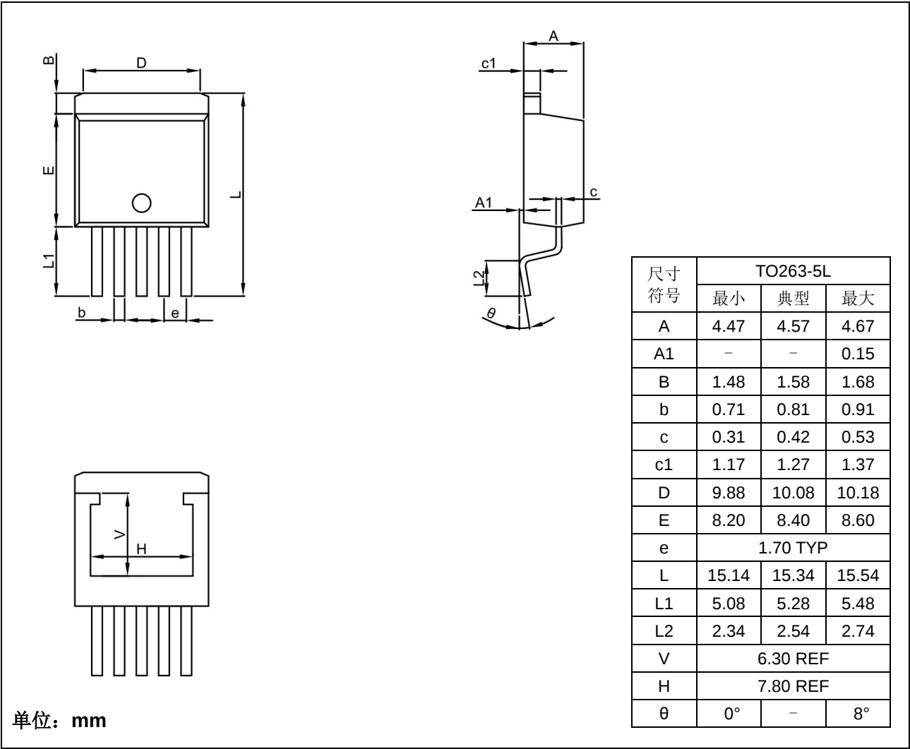
外形类型及尺寸图
