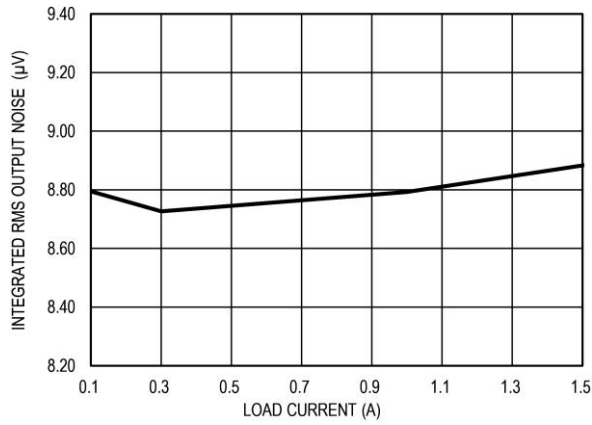
图 17 积分 RMS 输出噪声 ( V_{IN} = 5V , V_{OUT} = 3.3V )
