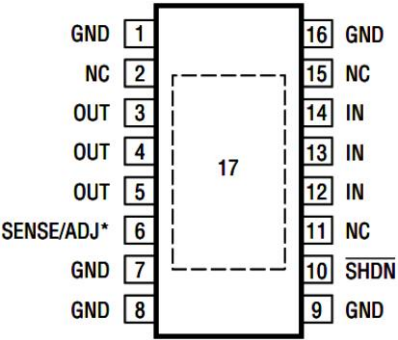
图 3 eTSSOP-16L 引脚配置
