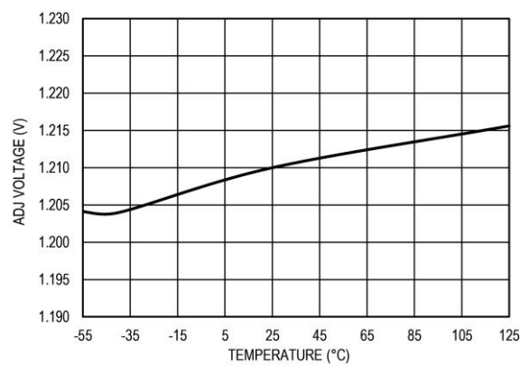
图 12 ADJ 引脚电压精度
