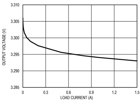
图 10 3.3V 输出电压 VS 负载电流
