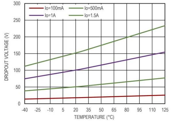
图 6 压差电压 VS 温度
