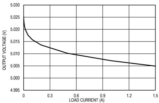
图 11 5.0V 输出电压 VS 负载电流
