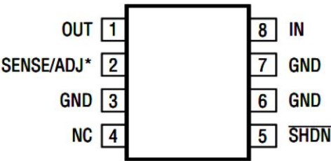
图 2 SOP-8L 引脚图
