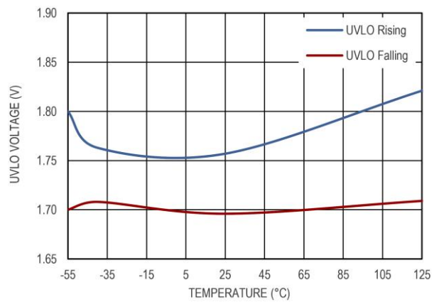
图 15 U_{VLO} 阈值
