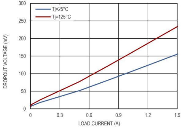
图 5 压差电压 VS 负载电流
