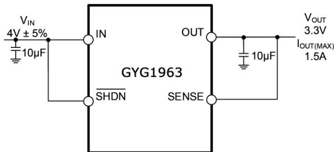
图 21 典型应用
