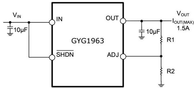
图 22 由外部电阻决定的输出电压
