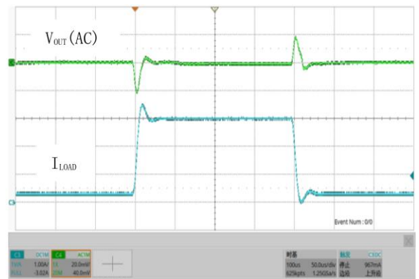
图 20 负载瞬态响应 ( V_{IN} = 2.8V , V_{OUT} = 1.8V , I_{OUT} = 0.1A \sim 1.5A )
