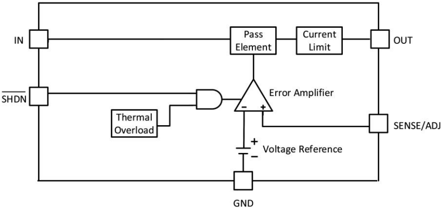
图 4 内部功能框图
