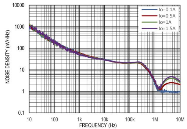
图 16 输出噪声谱密度 ( V_{IN} = 5V , V_{OUT} = 3.3V )
