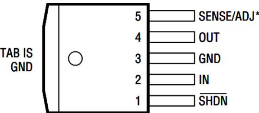
图 1 TO263-5L 引脚图
