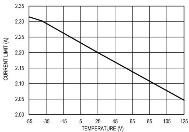
图 13 输出限流值 VS 温度
