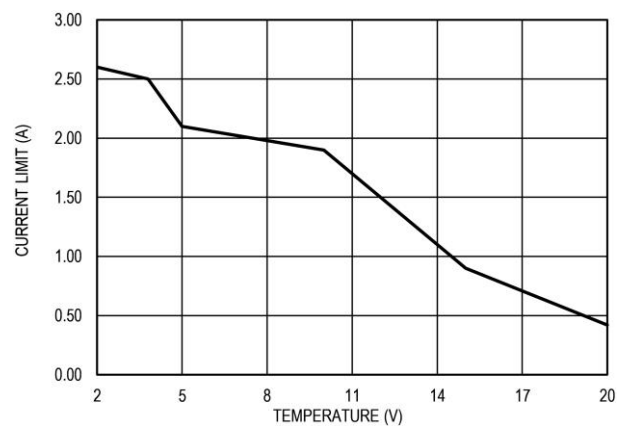
图 14 输出限流值 VS 输入输出压差
