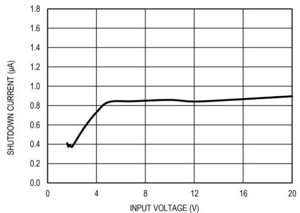
图 8 关机电流 VS 输入电压
