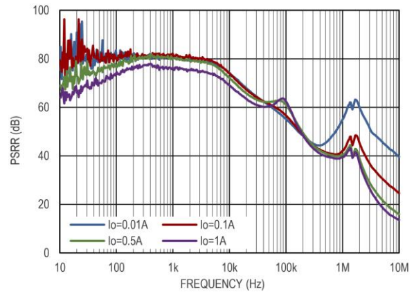
图 18 电源电压纹波抑制比 ( V_{IN} = 5V , V_{OUT} = 3.3V )
