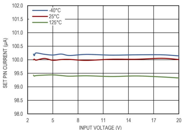
图 7 SET pin 电流和输入电压的关系
