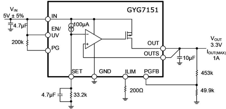
图 25 典型应用
