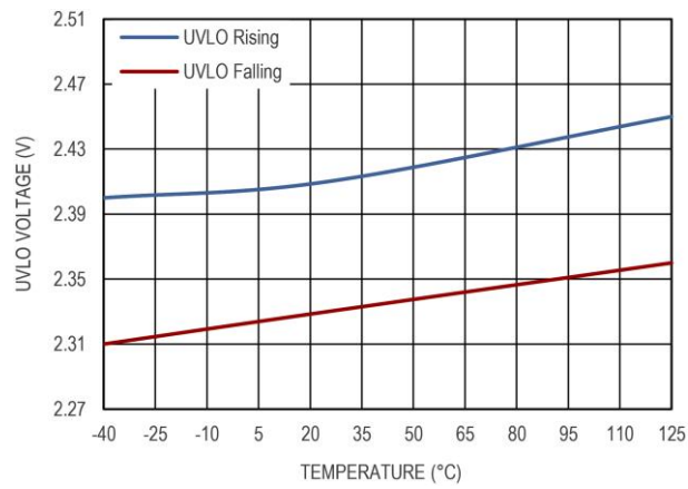
图 16 UVLO 阈值
