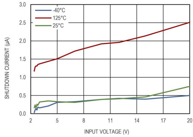
图 14 停机静态电流和输入电压的关系
