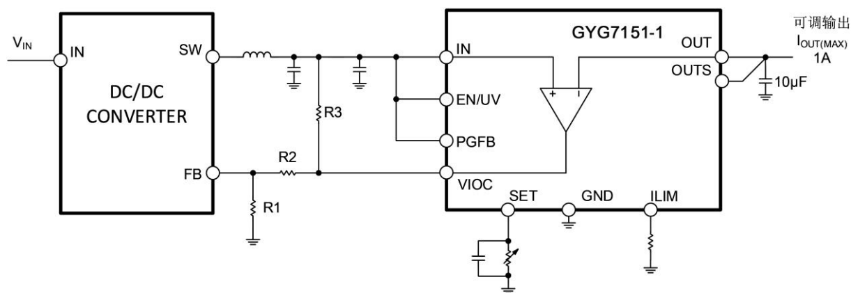
图 27 V_{IOC} 典型应用
