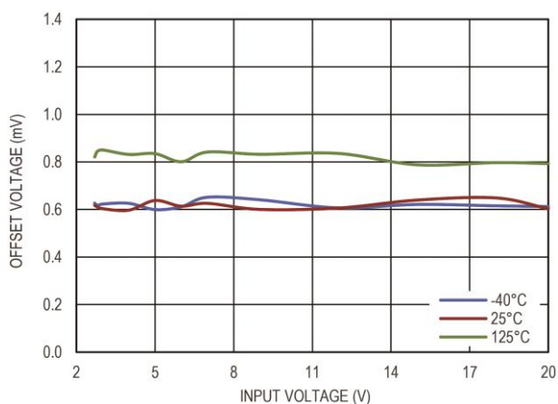
图 9 |V_{OUT}-V_{SET}| 和输入电压的关系, V_{OUT} = 1.8V
