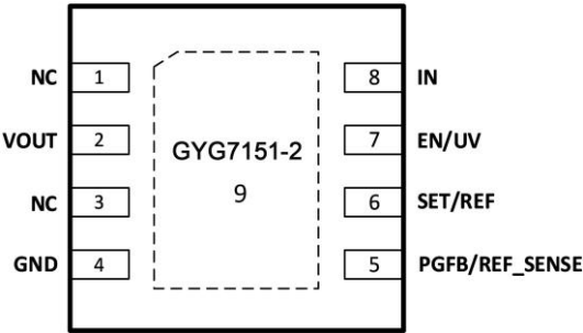
图 6 GYG7151-2 引脚图（顶视图）
