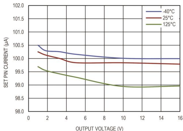
图 8 SET pin 电流和输出电压的关系
