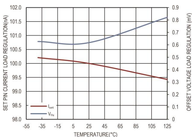
图 11 SET pin 电流和温度的关系
