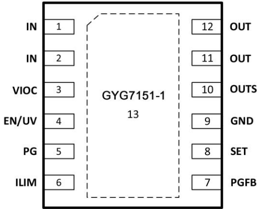
图 5 GYG7151-1 引脚图（顶视图）
