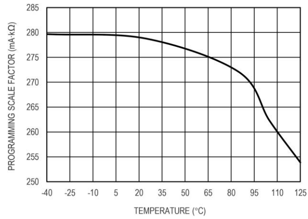
图 18 输出限流值编程因子
