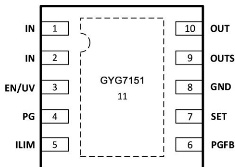
图 4 GYG7151 引脚图 (顶视图)
