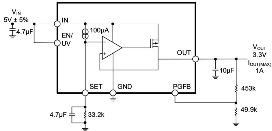
图 29 GYG7151-2 典型应用
