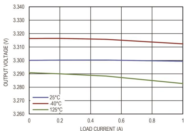
图 12 V_{OUT} = 3.3V 时的负载调整率
