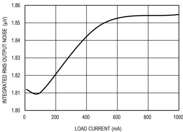
图 21 积分 RMS 输出噪声, V_{IN} = 5V , V_{OUT} = 3.3V
