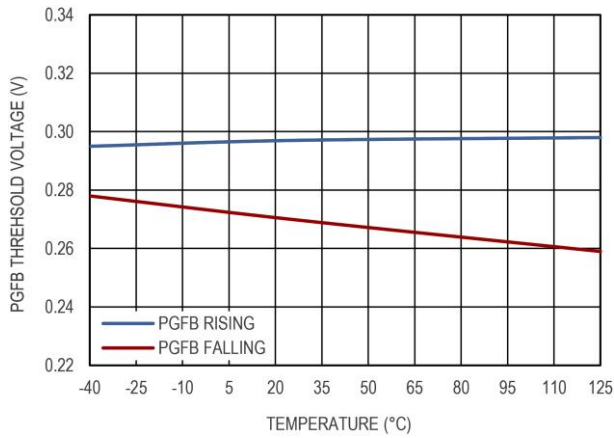
图 19 PGFB pin 阈值
