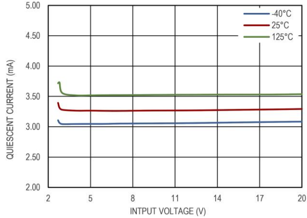
图 13 静态电流和输入电压的关系, I_{OUT} = 10\text{mA}
