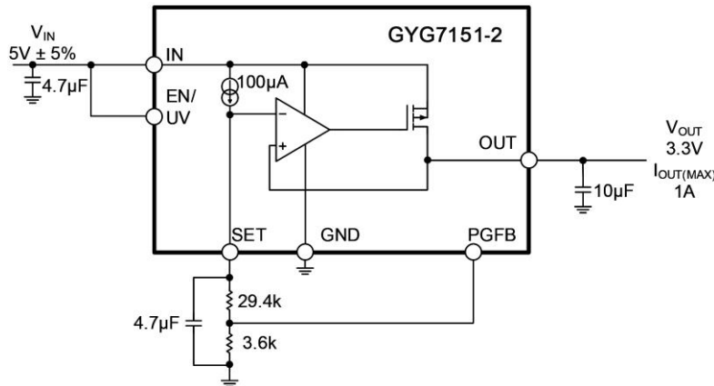
图 26 兼容 ADM7151 应用
