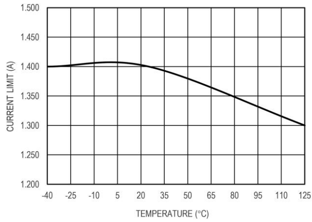
图 17 输出限流值和温度的关系
