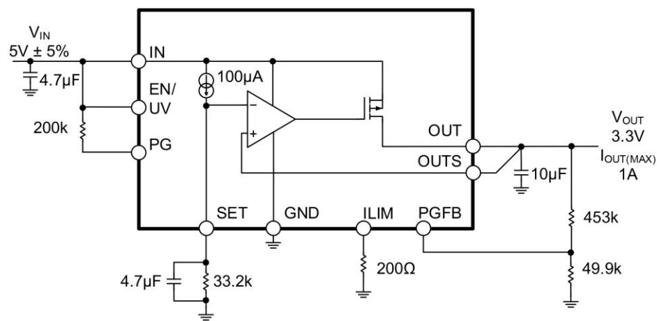
图 28 GYG7151、GYG7151-1 典型应用
