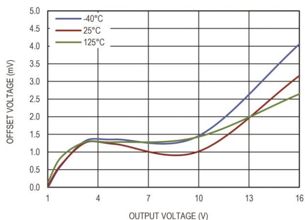
图 10 |V_{OUT}-V_{SET}| 和输出电压的关系
