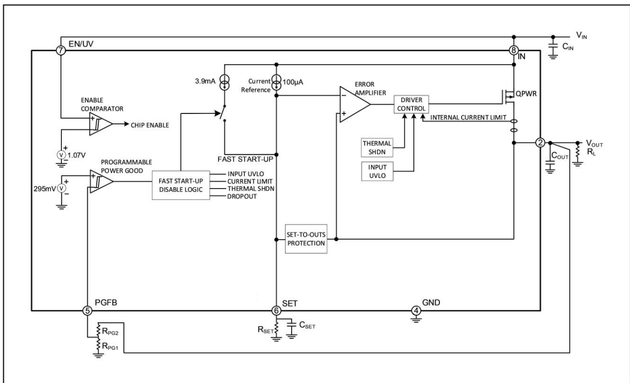
图 3 GYG7151-2 功能框图
