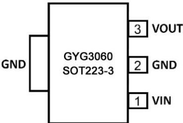
图 6 SOT223-3 引脚图
