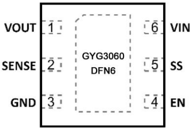
图 3 DFN6 引脚图
