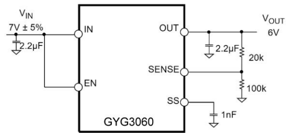
图 2 5V 可调输出至 6V
