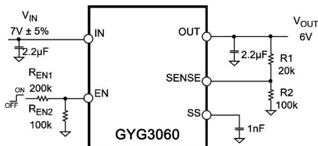
图 30 EN 引脚的典型分压器
