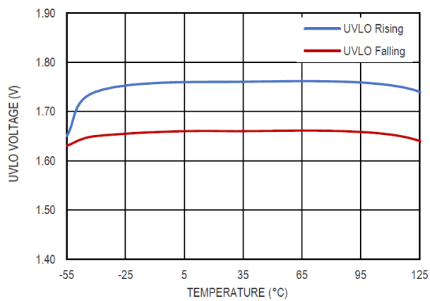
图 19 UVLO 阈值和温度的关系
