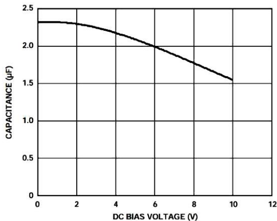
图 28 电容与电压关系特性
