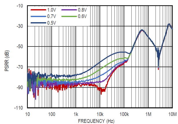
图 22 电源电压纹波抑制比与压差的关系, V_{OUT} = 5.0V
