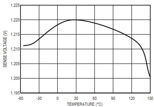
图 17 1.22V SENSE 引脚电压精度
