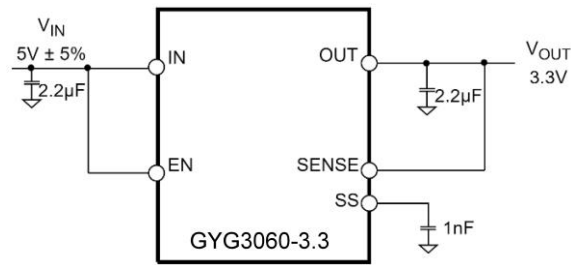
图 1 固定输出 3.3V
