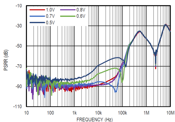
图 21 电源电压纹波抑制比与压差的关系, V_{OUT} = 3.3V
