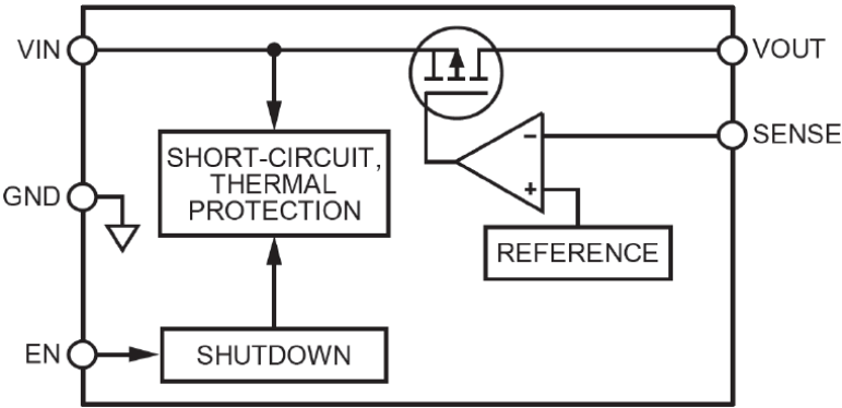
图 8 内部功能框图
