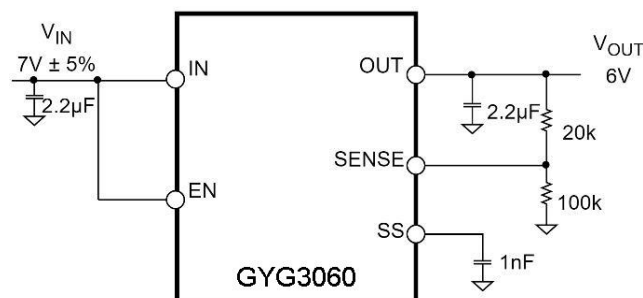
图 27 典型可调输出电压应用原理图
