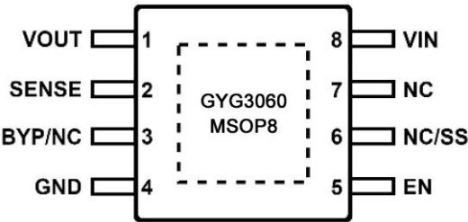
图 7 MSOP8 引脚图
