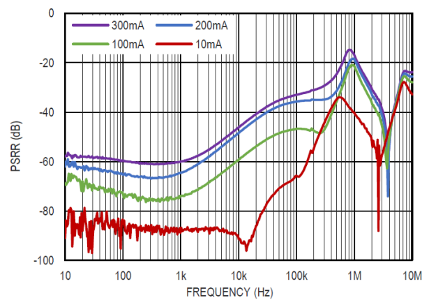
图 24 电源电压纹波抑制比与负载的关系, V_{OUT} = 5.0V
