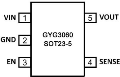
图 5 SOT23-5 引脚图
