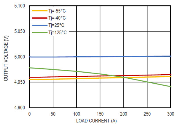
图 15 5.0V 输出电压和负载电流的关系
