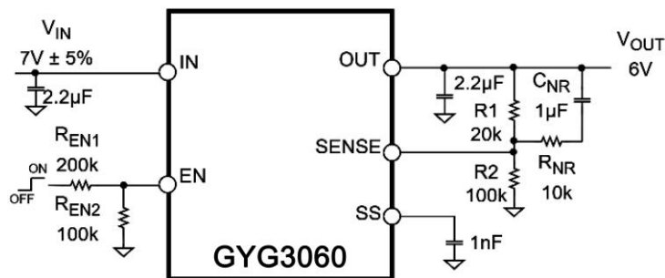
图 31 噪声优化
