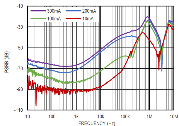
图 23 电源电压纹波抑制比与负载的关系, V_{OUT} = 3.3V
