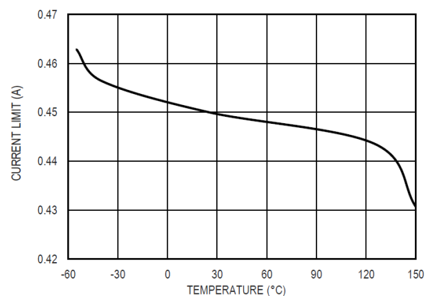
图 18 输出限流值和温度的关系
