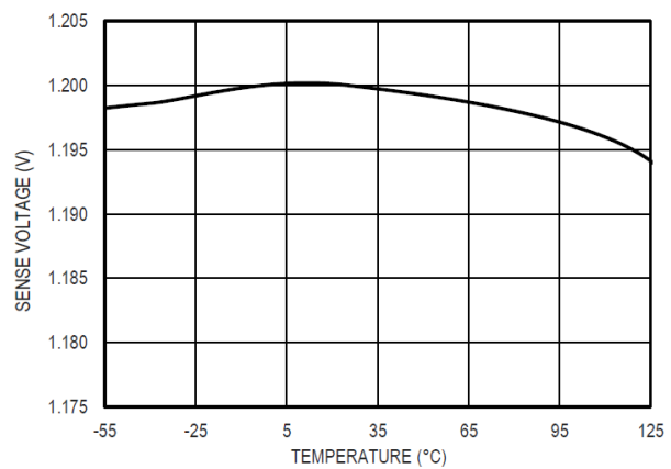
图 16 1.2V SENSE 引脚电压精度
