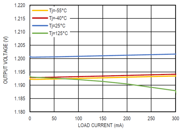
图 13 1.2V 输出电压和负载电流的关系
