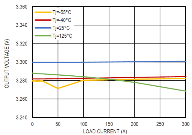
图 14 3.3V 输出电压和负载电流的关系
