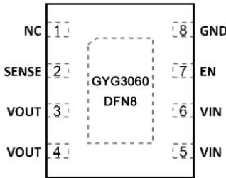
图 4 DFN8 引脚图
