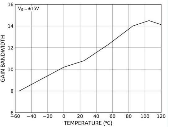
图 8 增益带宽积随温度的变化
