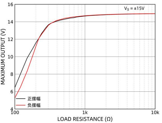
图 10 最大输出电压随负载阻抗的变化
