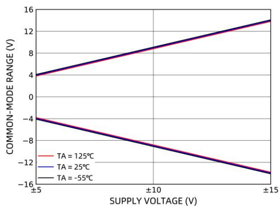
图 17 共模电压范围随电源电压的变化
