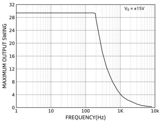
图 9 最大输出摆幅
