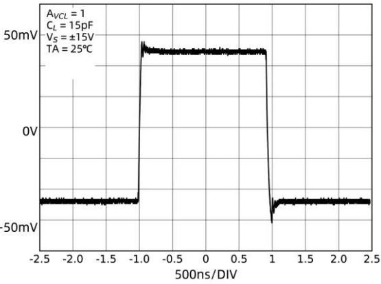
图 13 小信号瞬态响应
