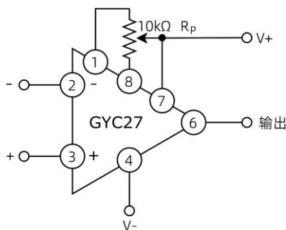
图 20 失调归零电路
