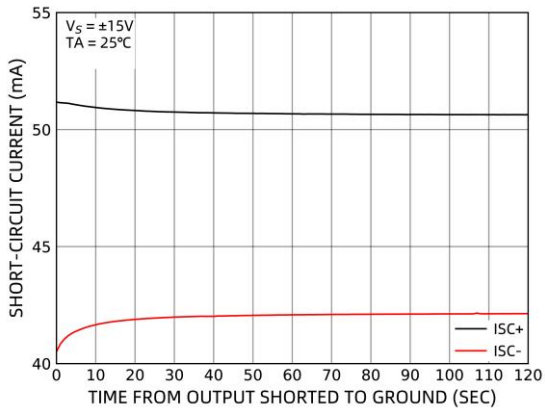
图 15 短路电流随时间的变化
