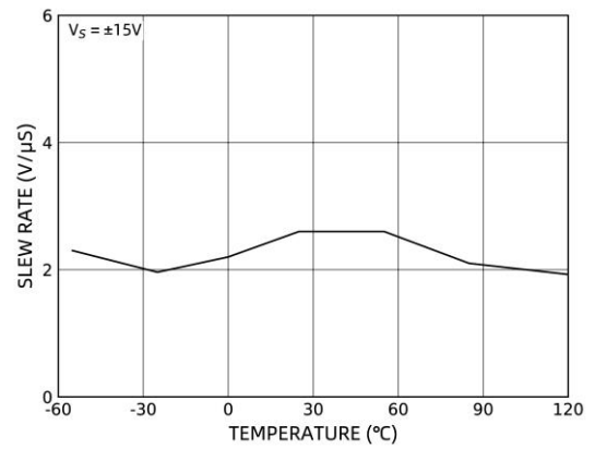
图 7 压摆率随温度的变化
