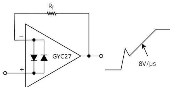
图 22 阶跃响应
