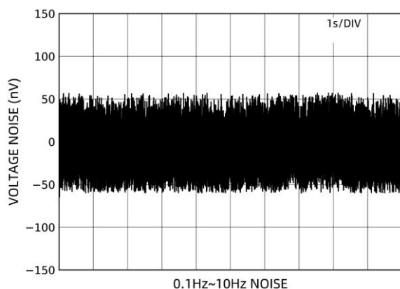
图 19 低频噪声
