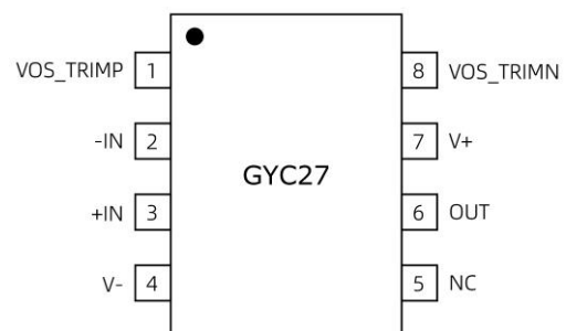
管脚示意图
