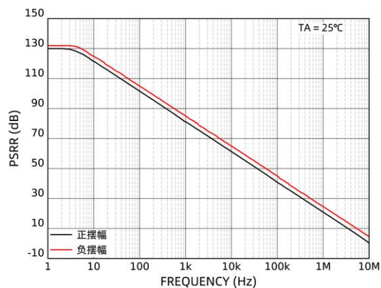
图 18 PSRR
