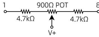
图 21 失调电压调整
