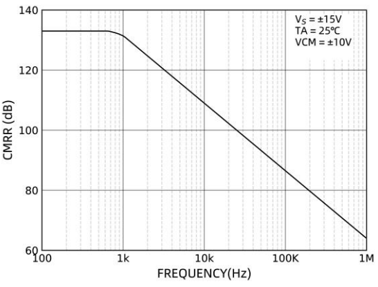
图 16 CMRR
