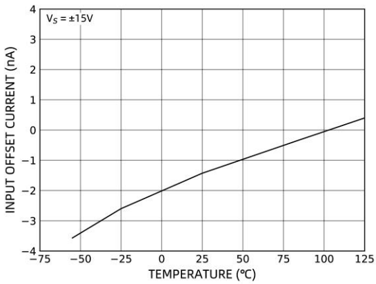
图 5 输入失调电流随温度的变化
