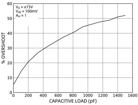
图 11 小信号过冲随容性负载的变化
