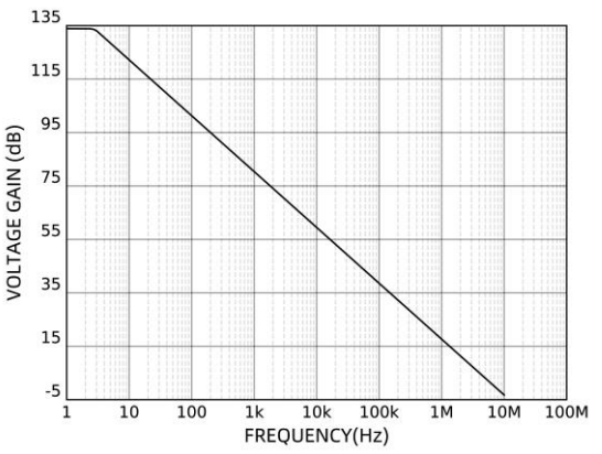
图 6 电压增益
