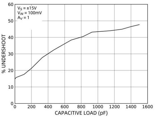
图 12 小信号预冲随容性负载的变化
