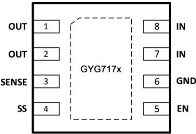
图 1 DFN-8L 引脚图（裸露焊盘必须焊接到 PCB 上）
