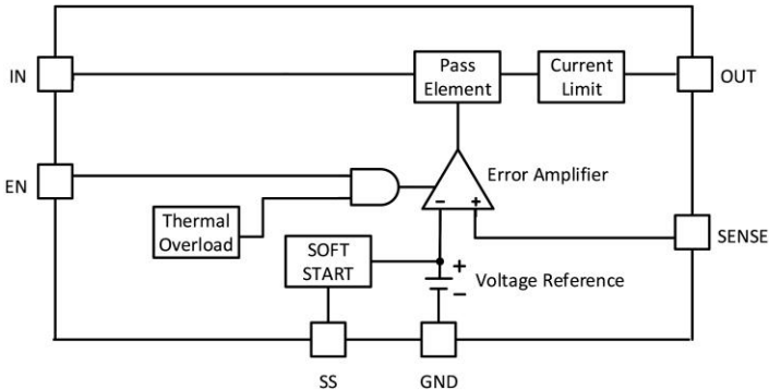
图 2 内部功能框图
