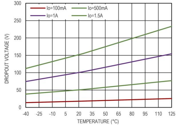
图 4 压差电压 VS 温度
