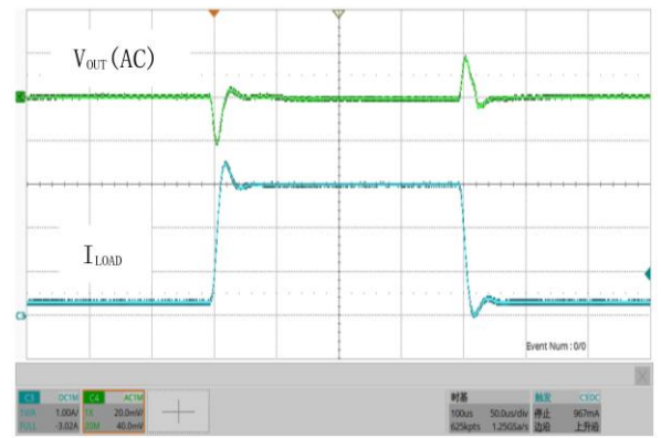
图 18 负载瞬态响应 ( V_{IN} = 2.8V , V_{OUT} = 1.8V , I_{OUT} = 0.1A \sim 1.5A )
