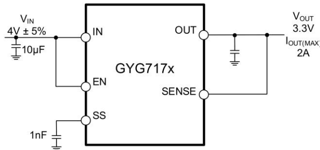
图 19 典型应用
