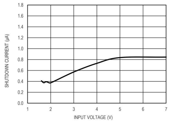
图 6 关机电流 VS 输入电压
