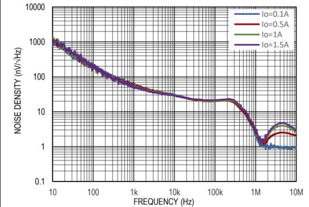
图 14 输出噪声谱密度 ( V_{IN} = 5V , V_{OUT} = 3.3V )
