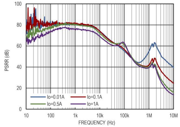
图 16 电源电压纹波抑制比 ( V_{IN} = 5V , V_{OUT} = 3.3V )
