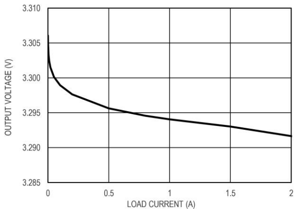
图 8 3.3V 输出电压 VS 负载电流
