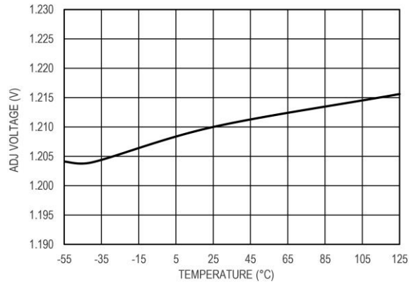
图 10 SENSE 引脚电压精度
