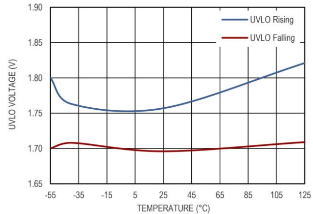
图 13 U_{VLO} 阈值
