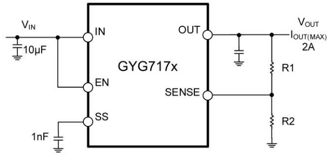
图 20 由外部电阻决定的输出电压
