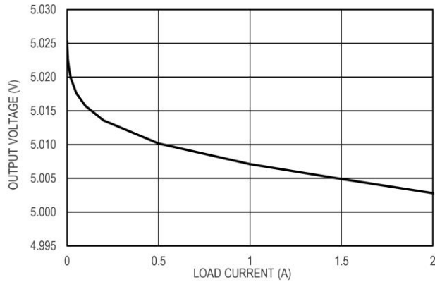
图 9 5.0V 输出电压 VS 负载电流
