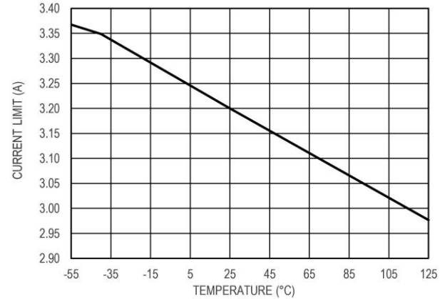
图 11 输出限流值 VS 温度
