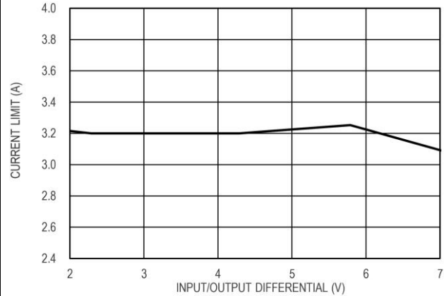
图 12 输出限流值 VS 输入输出压差
