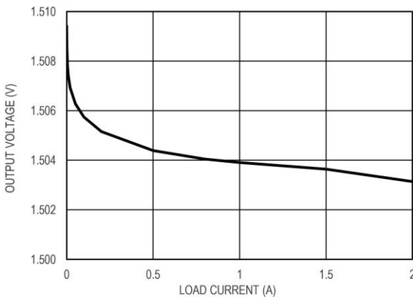
图 7 1.5V 输出电压 VS 负载电流
