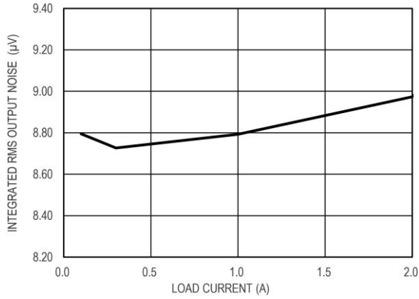
图 15 积分 RMS 输出噪声 ( V_{IN} = 5V , V_{OUT} = 3.3V )
