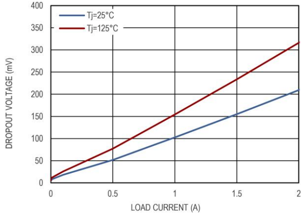
图 3 压差电压 VS 负载电流
