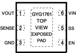
图 4 DFN-6L 引脚图
