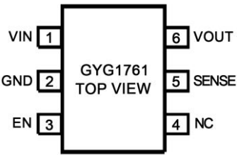
图 5 SOT23-6L 引脚图
