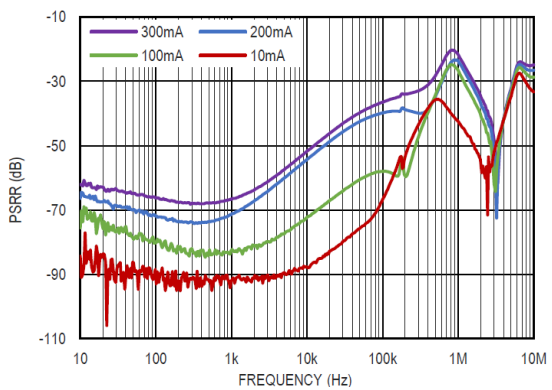
图 21 电源电压纹波抑制比与负载的关系, V_{OUT} = 3.3V
