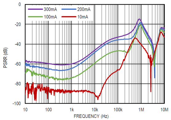
图 22 电源电压纹波抑制比与负载的关系, V_{OUT} = 5.0V
