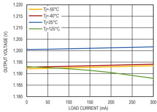
图 11 1.2V 输出电压和负载电流的关系
