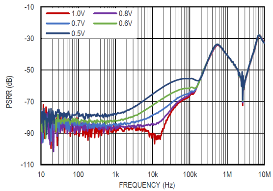
图 20 电源电压纹波抑制比与压差的关系, V_{OUT} = 5.0V
