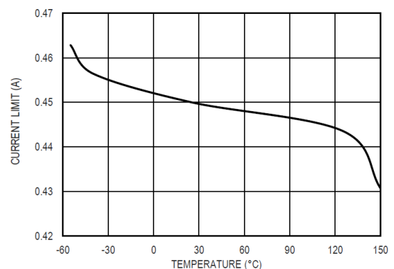
图 16 输出限流值和温度的关系
