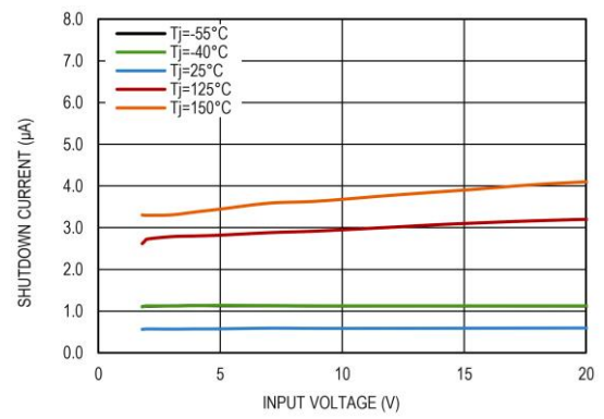
图 10 关机电流和输入电压的关系
