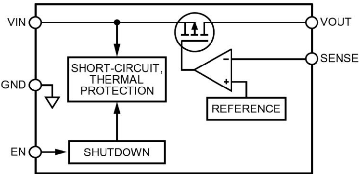
图 3 内部功能框图
