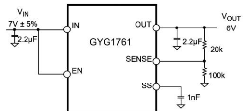
图 2 5V 可调输出至 6V
