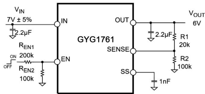
图 28 EN 引脚的典型分压器
