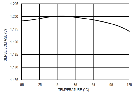
图 14 1.2V SENSE 引脚电压精度
