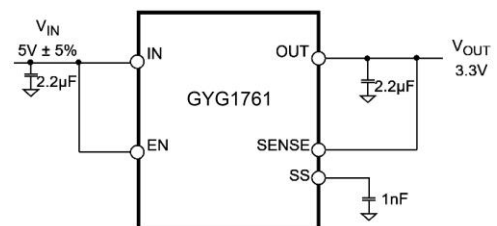
图 1 固定输出 3.3V
