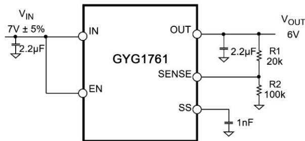
图 25 典型可调输出电压应用原理图
