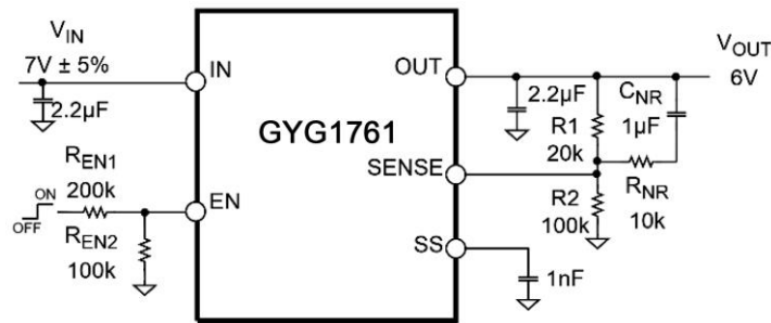
图 29 噪声优化
