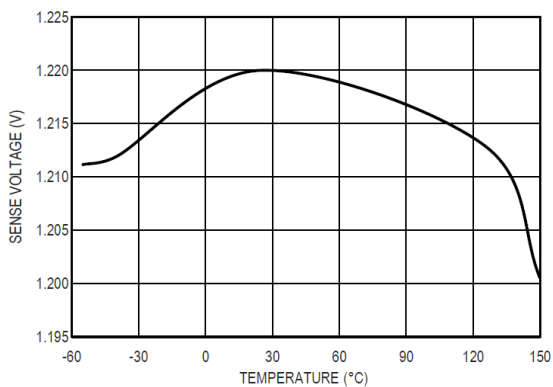
图 15 1.22V SENSE 引脚电压精度
