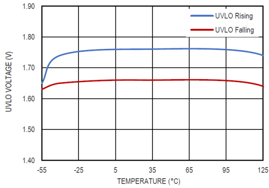
图 17 UVLO 阈值和温度的关系
