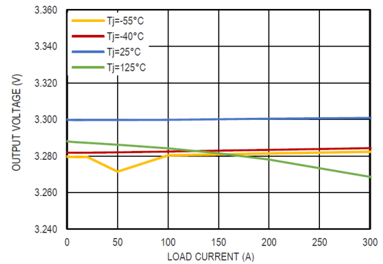
图 12 3.3V 输出电压和负载电流的关系
