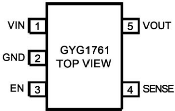
图 6 SOT23-5L 引脚图
