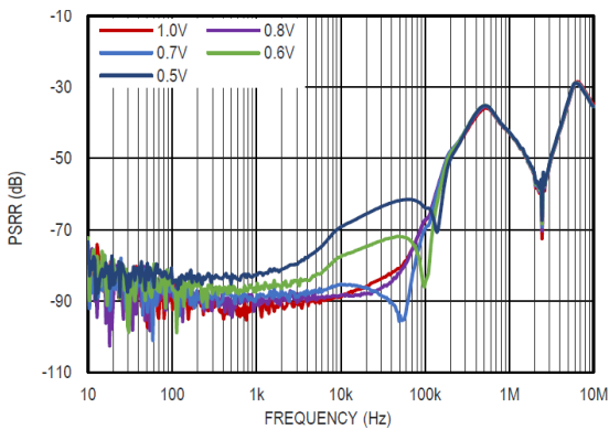
图 19 电源电压纹波抑制比与压差的关系, V_{OUT} = 3.3V
