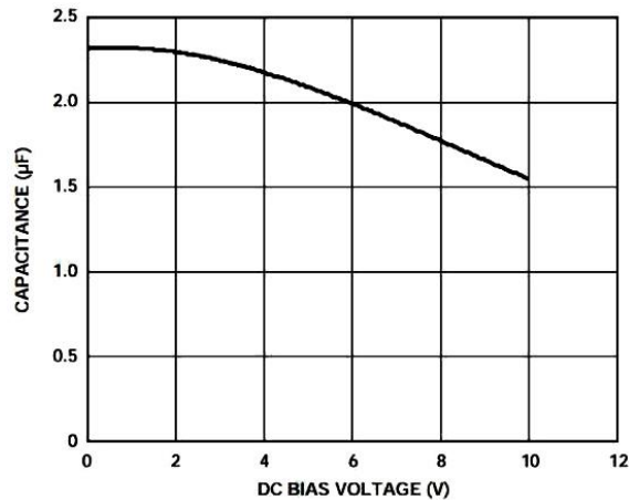
图 26 电容与电压关系特性
