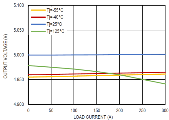
图 13 5.0V 输出电压和负载电流的关系
