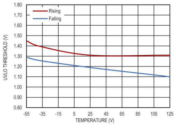
图 15 U_{VLO} 阈值，BIAS 浮空
