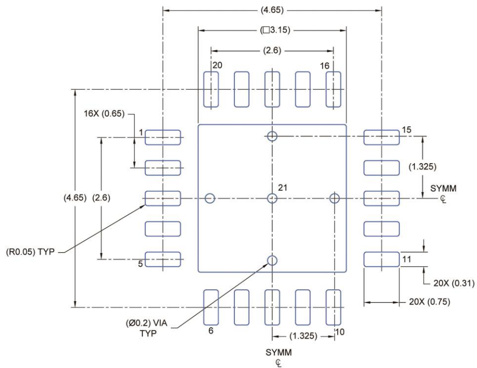
焊盘图纸 (比例: 15X)
