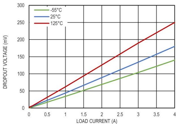
图 11 压差电压和负载的关系, V_{OUT} = 5.0\text{V} , BIAS 浮空
