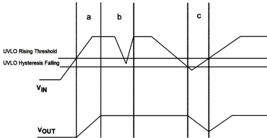
图 30 欠压锁定条件和输出变化
