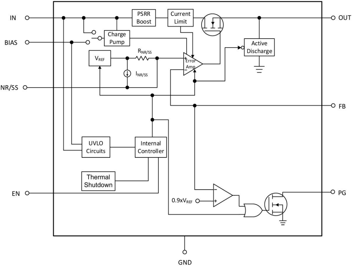
图 4 GYG74401-2A3 和 GYG74401-2B3 内部功能框图
