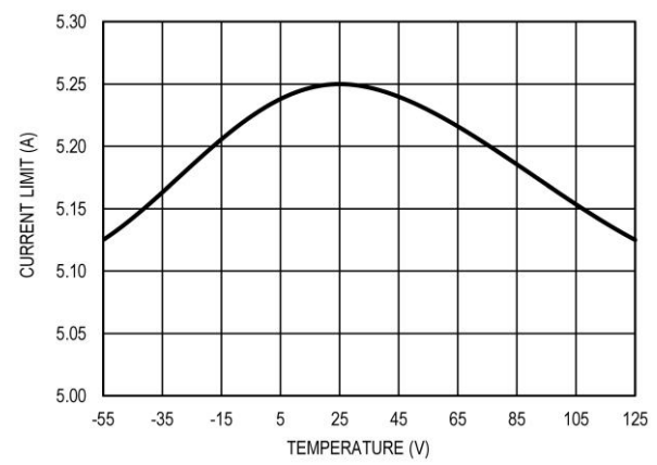
图 18 GYG74401 输出限流值和温度的关系 (4A)
