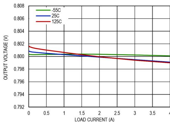
图26 负载调整率, BIAS浮空
