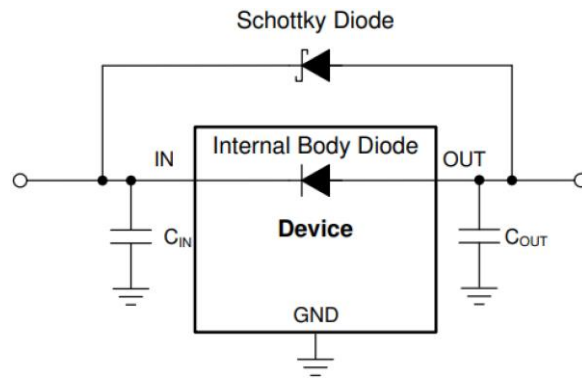
图 32 反向电流保护应用电路
