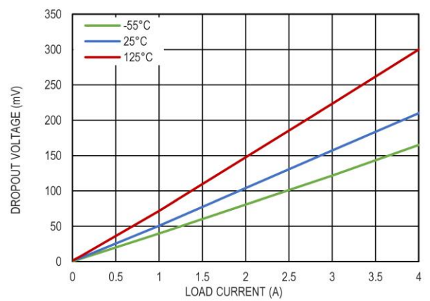
图 10 压差电压和负载的关系, V_{OUT} = 1.5\text{V} , BIAS 浮空
