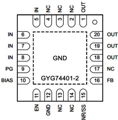
图 2 QFN20（5mm × 5mm）引脚图
