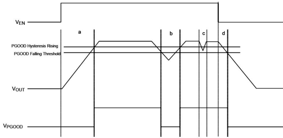
图 31 PG 触发场景具有不同的运行状态
