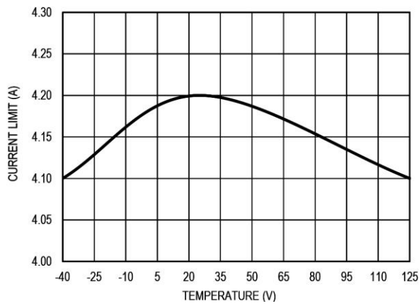
图 17 输出限流值和温度的关系 (3A)
