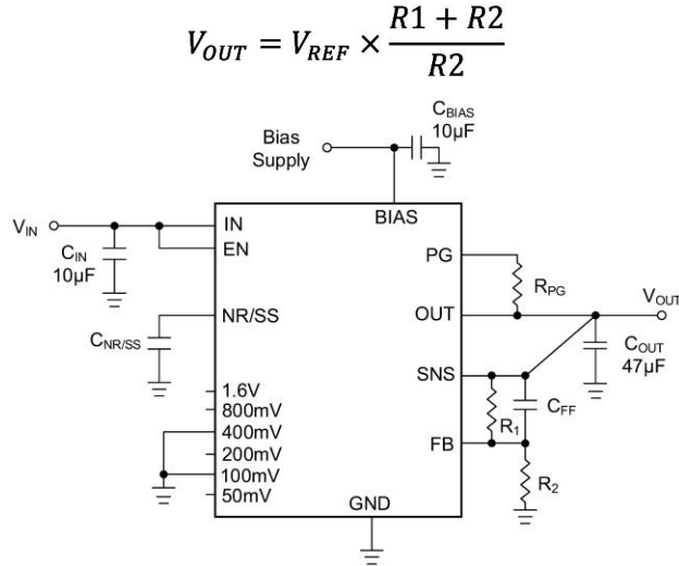
图 28 由外部电阻决定的输出电压
