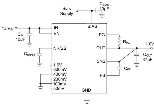
图5 GYG74401-1典型应用
