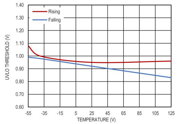
图 16 U_{VLO} 阈值， V_{BIAS} = 5V
