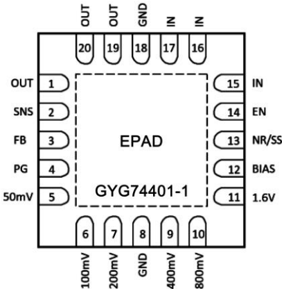
图 1 QFN20（3.5mm × 3.5mm）引脚图
