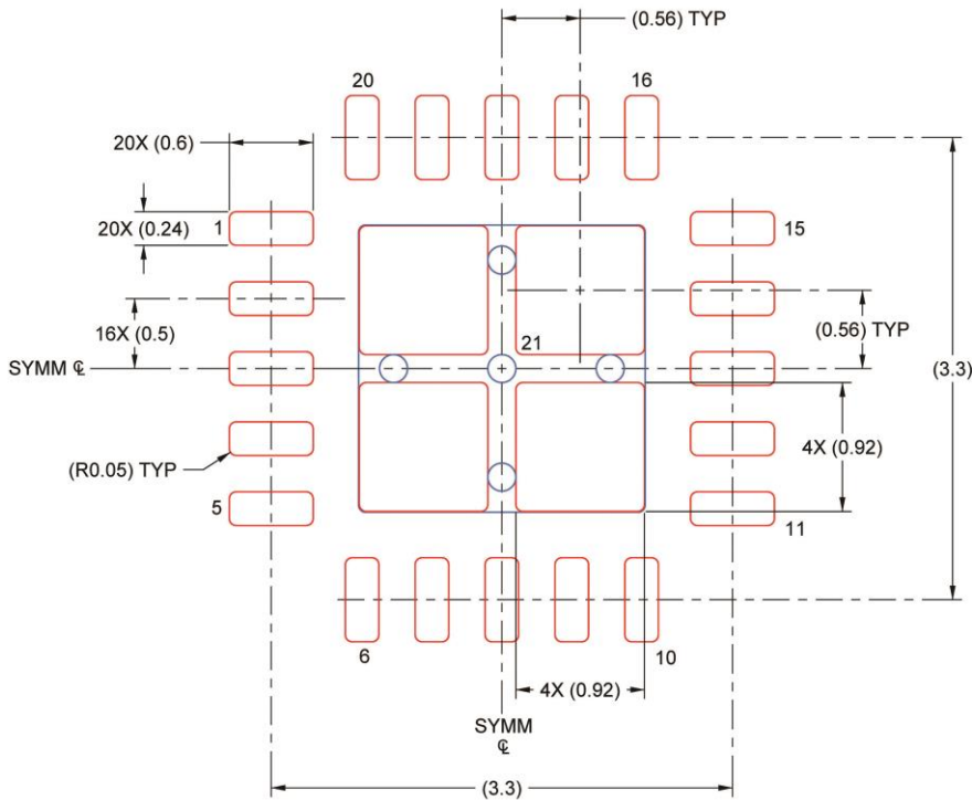
焊锡膏图纸
