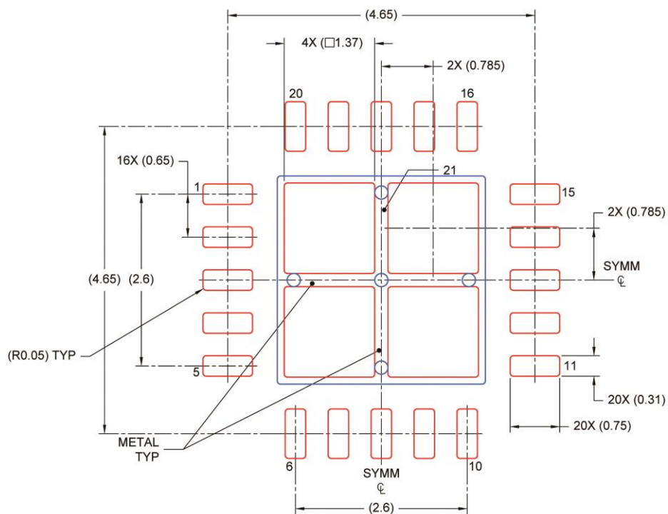
焊锡膏图纸
