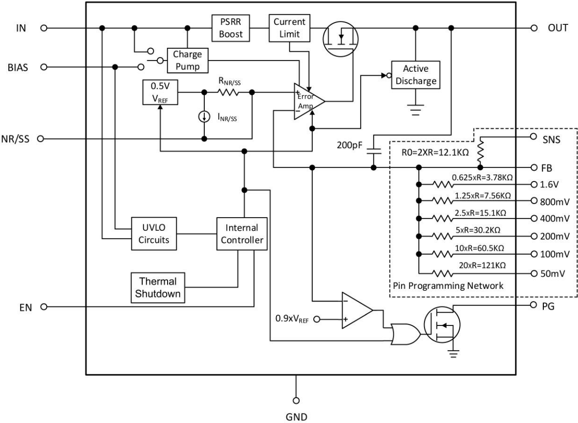
图 3 GYG74401-1A3 和 GYG74401-1B3 内部功能框图
