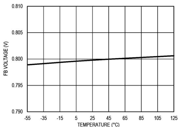
图25 FB引脚电压和温度的关系
