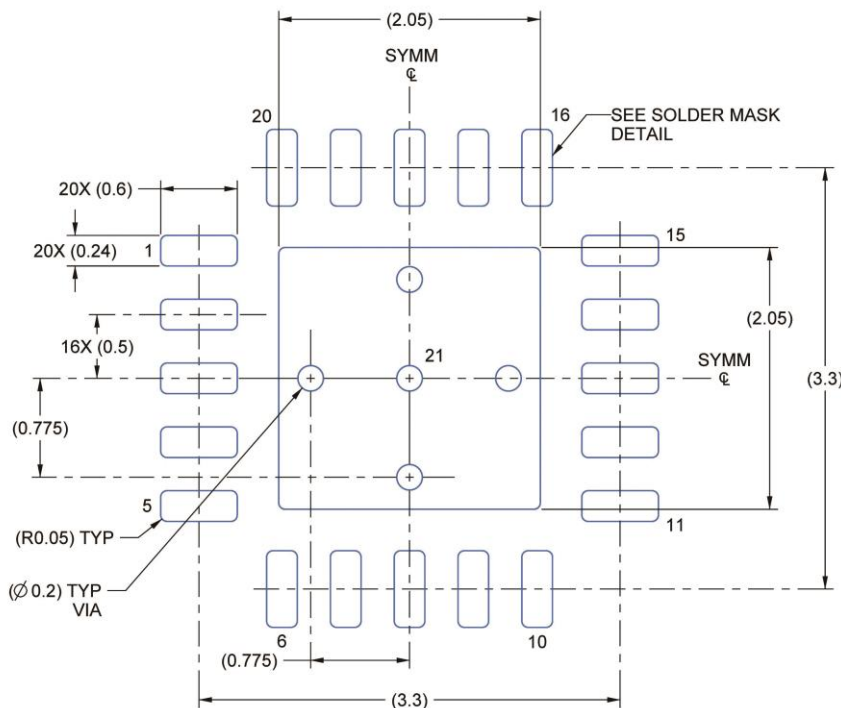
焊盘图纸 (比例: 20X)
