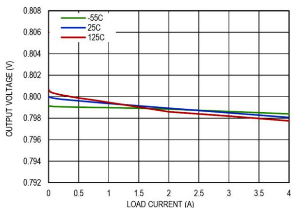
图27 负载调整率, V_{BIAS} = 5V
