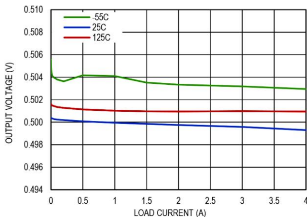
图 9 负载调整率, V_{BIAS} = 5\text{V}
