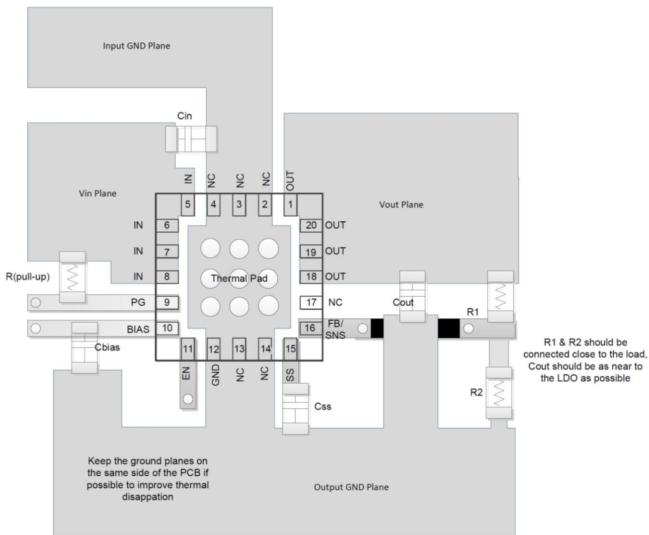
图 30 GYG74401-2 布局示例
