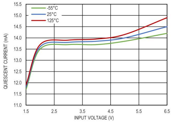
图 13 静态电流和输入电压的关系， I_{OUT} = 1mA
