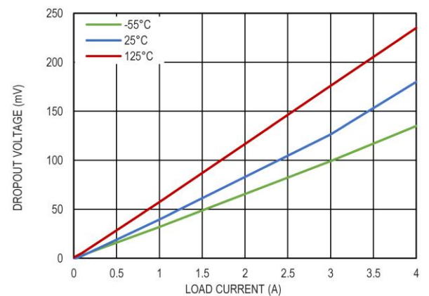
图 12 压差电压和负载的关系, V_{OUT} = 1.2\text{V} , V_{BIAS} = 5\text{V}
