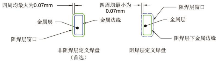
阻焊层信息
