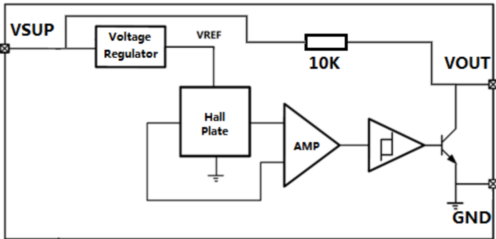
KM142F 功能框图
