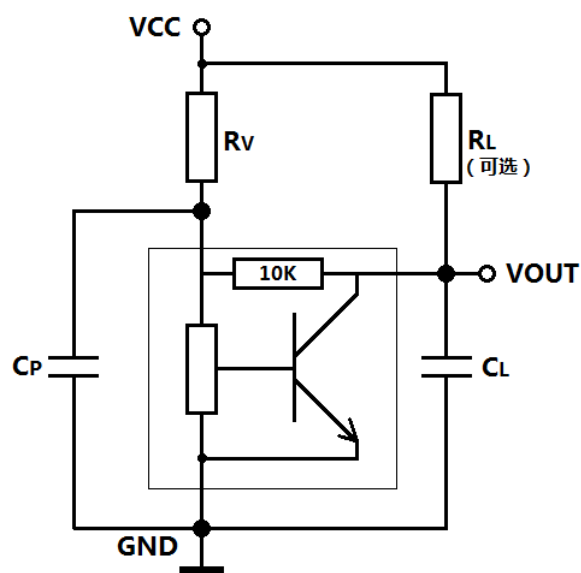
应用电路 2
