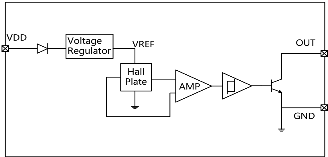
KM142H 功能框图
