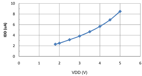
静态电流 vs. 工作电压
