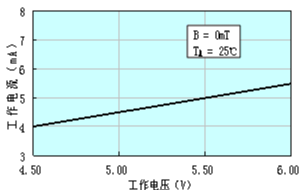
工作电流与工作电压关系曲线
