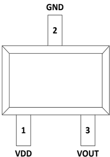
SOT23
