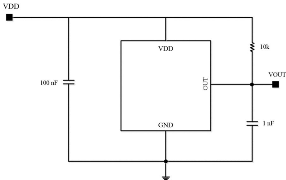
图 4 典型应用图
