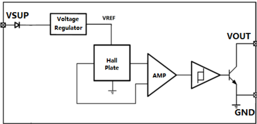
KM41F 功能框图
