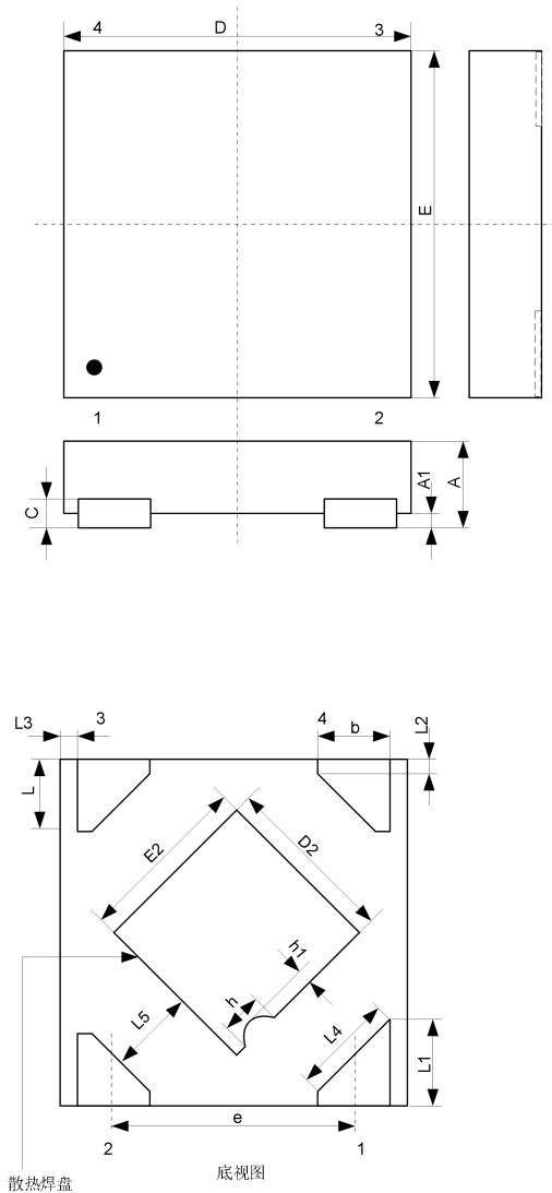
(3)DFN4L 封装
