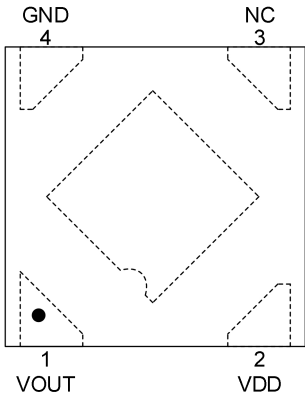
DFN4L 封装
