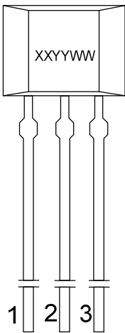
TO-92S 封装
