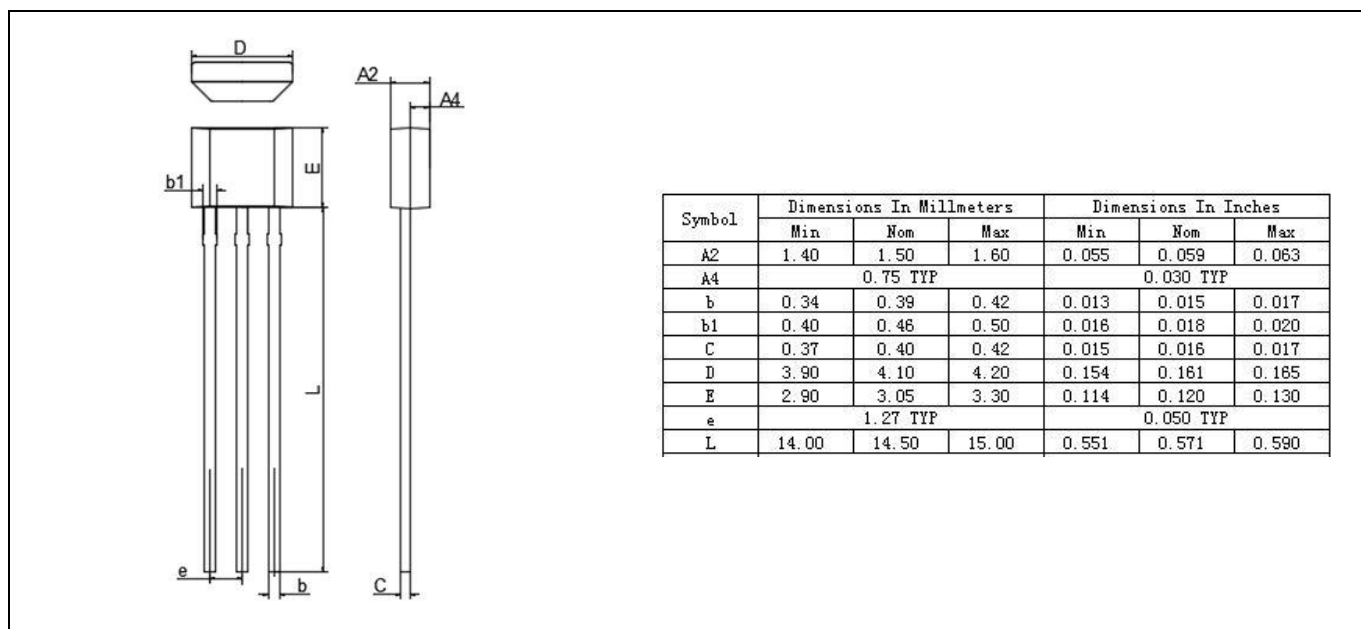
TO-92S 封装图
