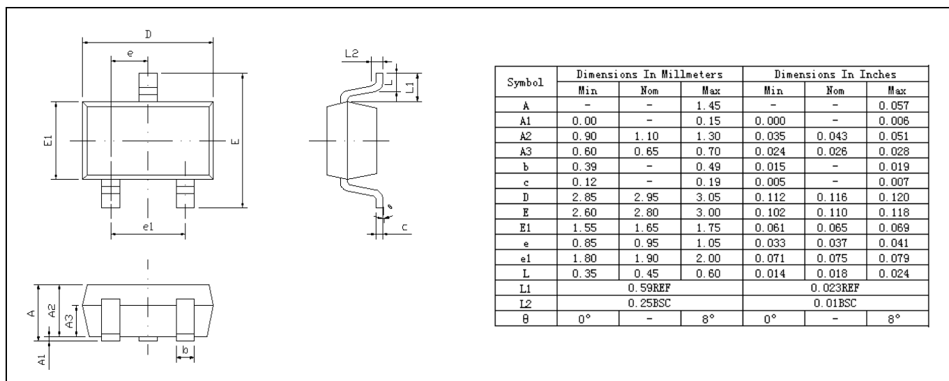
SOT23-3 封装图
