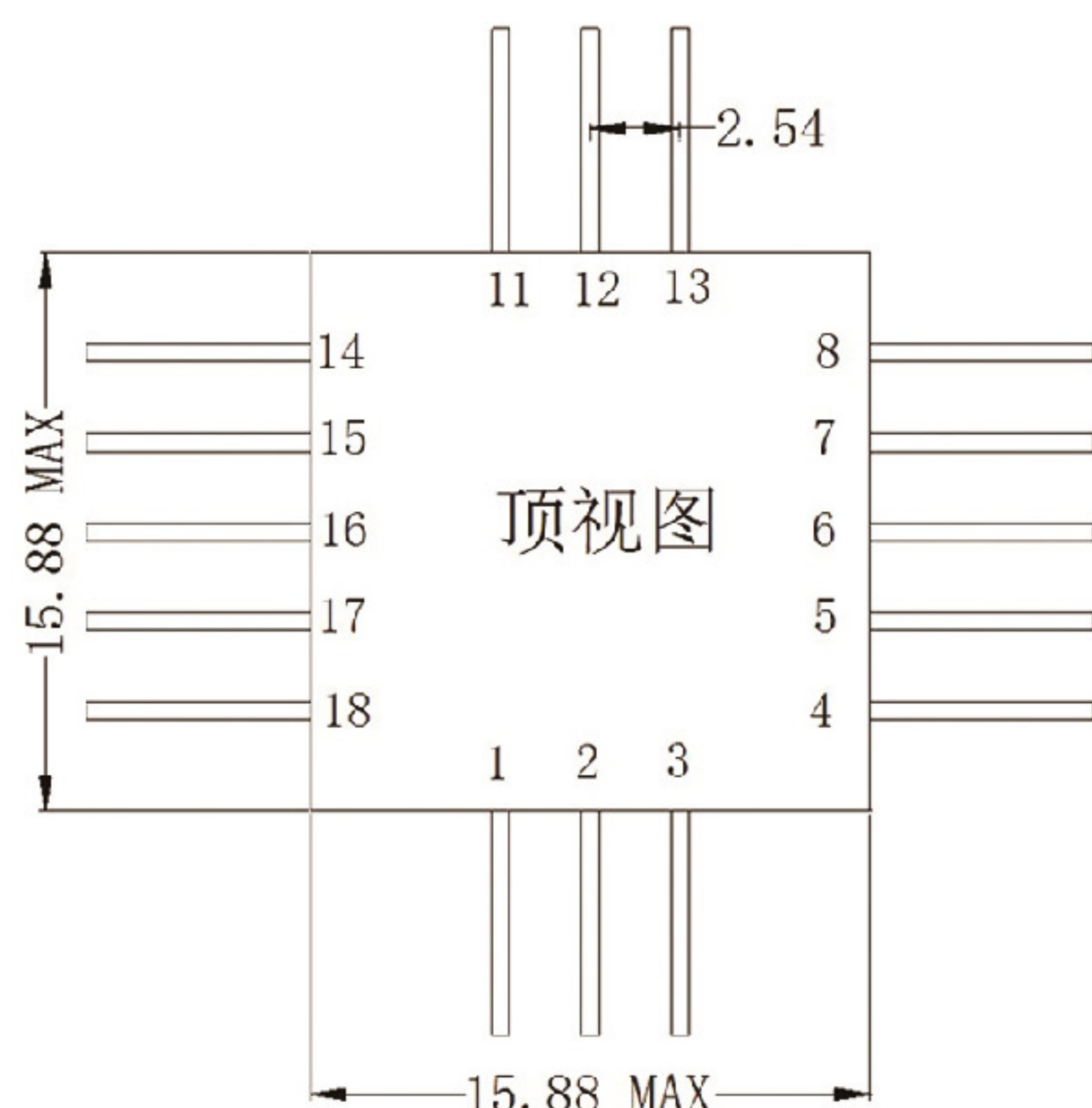
封装图
