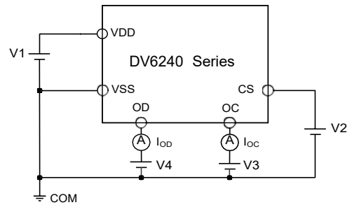
图 6: (测试电路 4)
