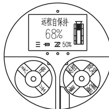
图 12 远程控制
