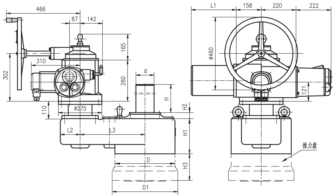
XFSND-Z350~XFSND-Z1000 外形尺寸
