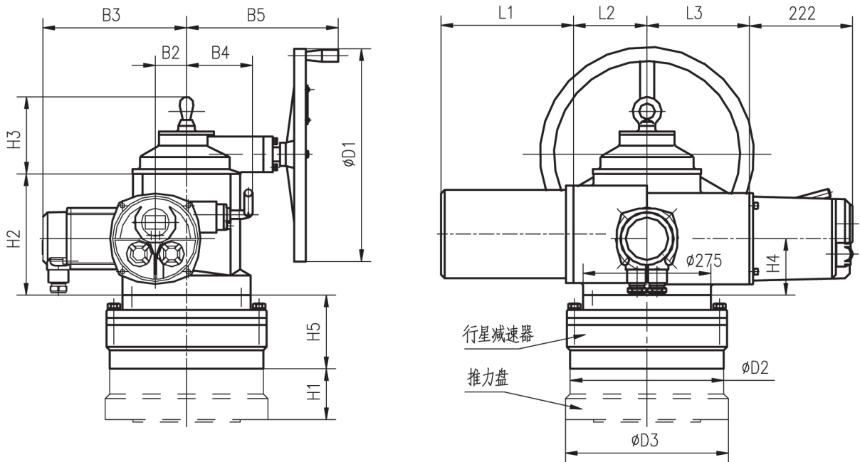
XFSND-Z90~XFSND-Z250 外形尺寸 (注: XFSND-Z 120 90 无行星减速器)
