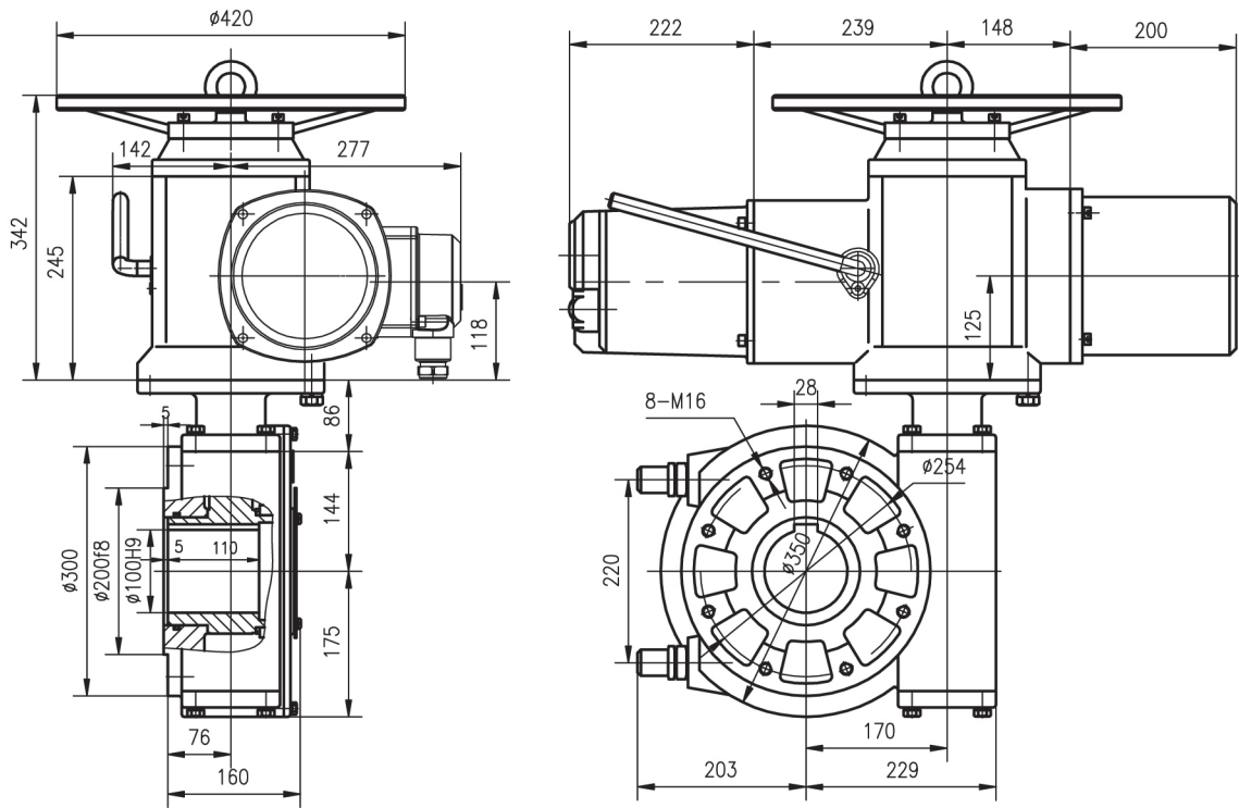
XFSND-DQ800和XFSND-DQ1000 外形和连接尺寸
