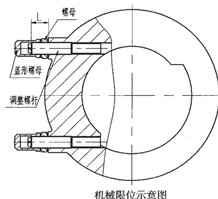
机械限位示意图
