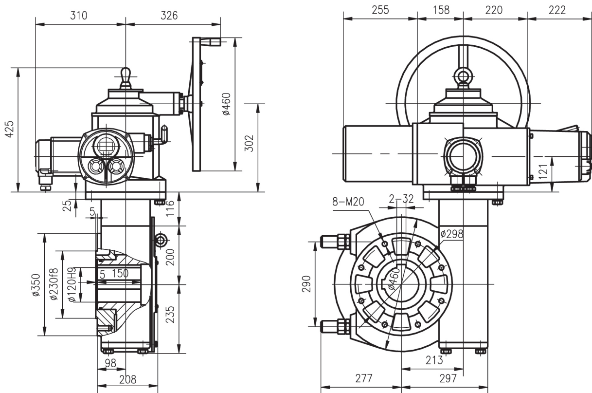
XFSND-DQ1600和XFSND-DQ2000 外形和连接尺寸
