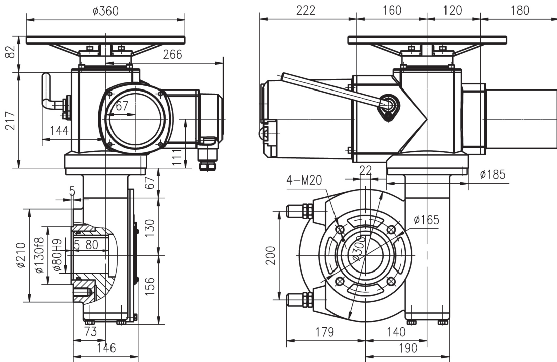
XFSND-DQ400 和 XFSND-DQ600 外形和连接尺寸
