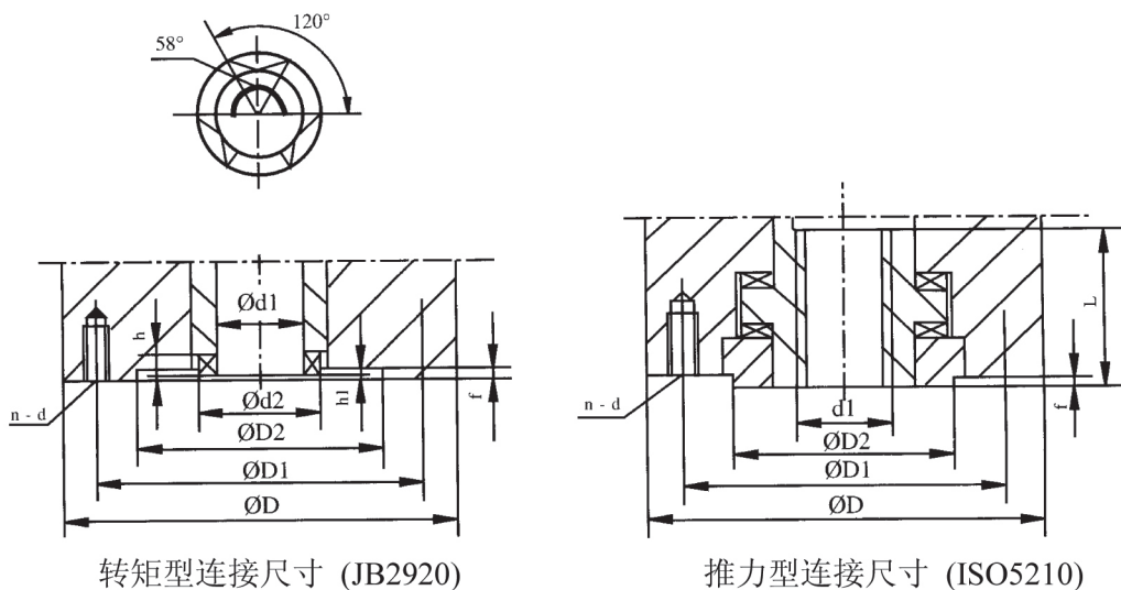
XFSND-Z 系列执行机构连接尺寸表
