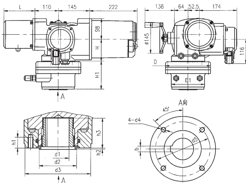
XFSND-Q 系列外形和连接尺寸图
