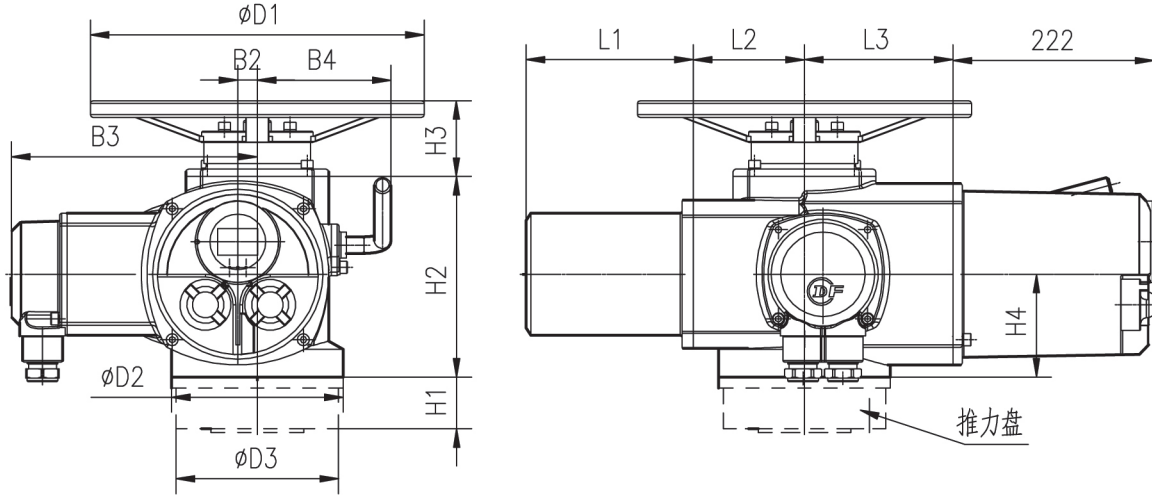
XFSND-Z5~XFSND-Z60 外形尺寸
