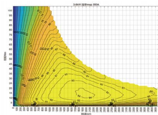
效率MAP
