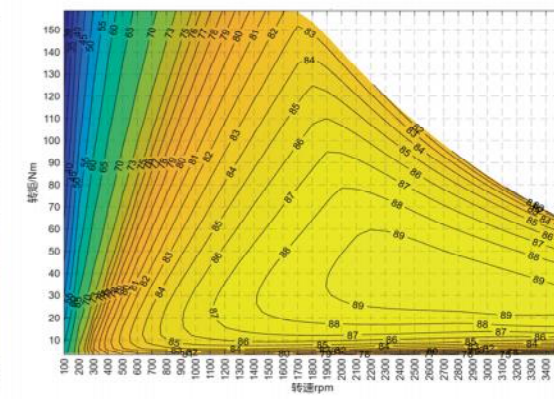
效率MAP
