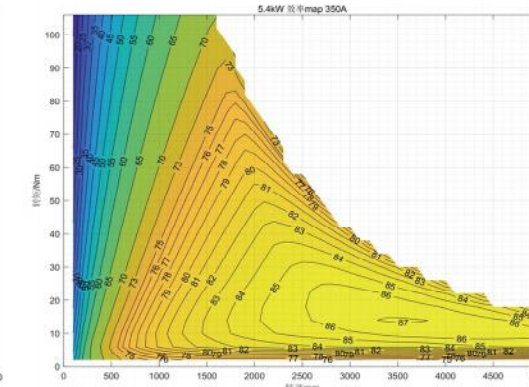
效率MAP
