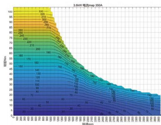
电流MAP
