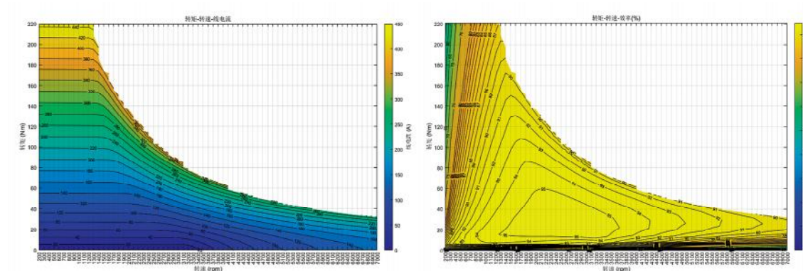
电流MAP
