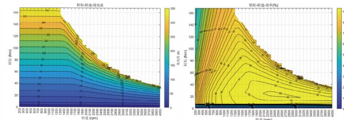
电流MAP
