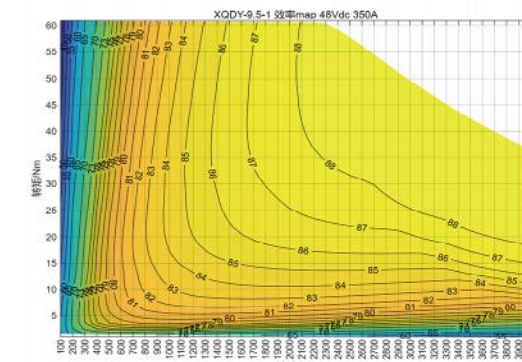
效率MAP
