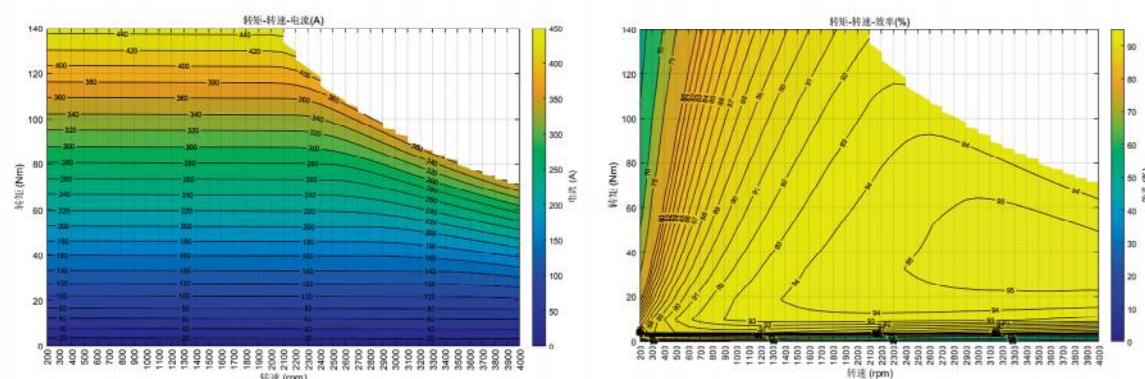
电流MAP
