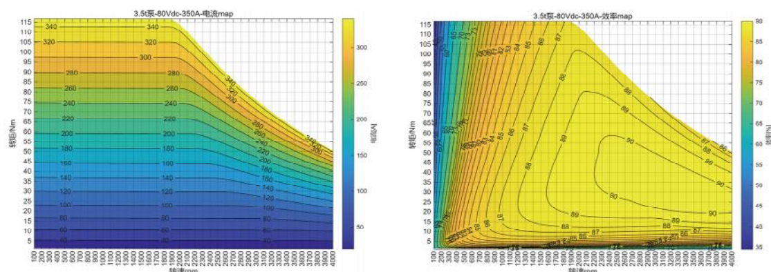
电流MAP
