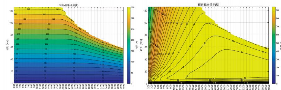
电流MAP
