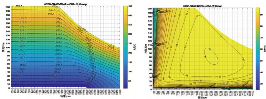
电流MAP
