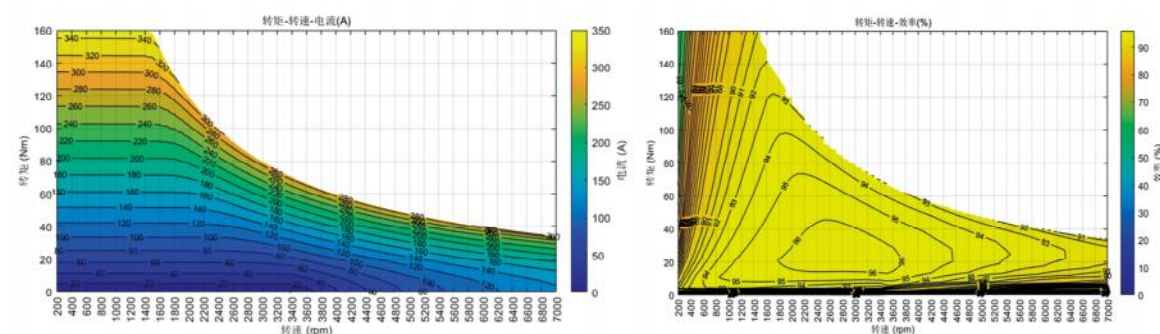
电流MAP
