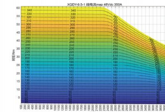
电流MAP
