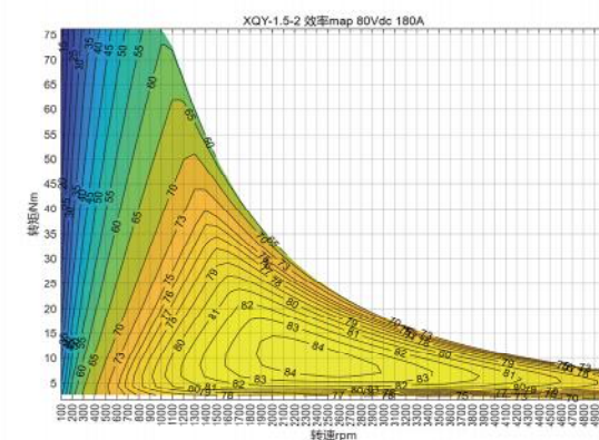
效率MAP
