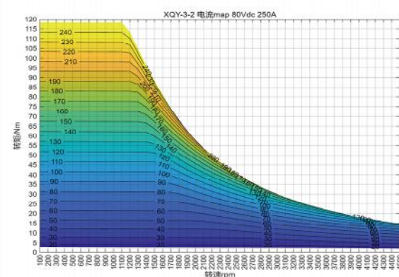
电流MAP
