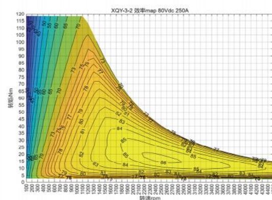
效率MAP
