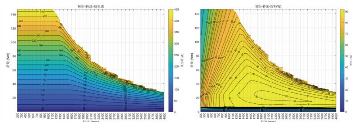
电流MAP
