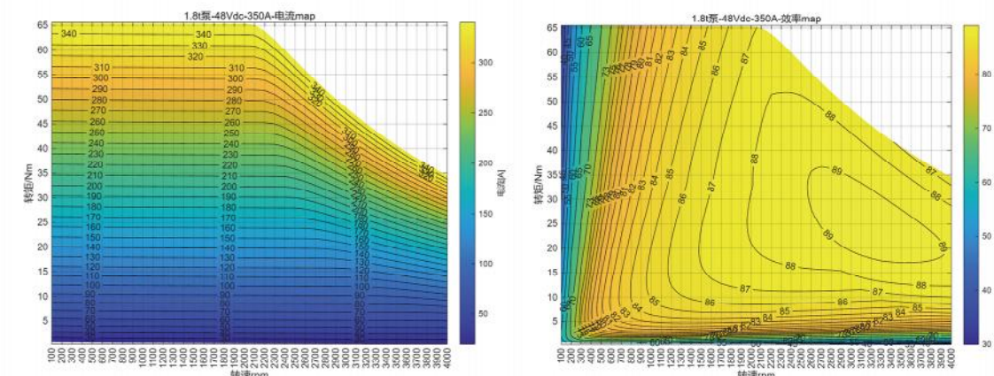
效率MAP
