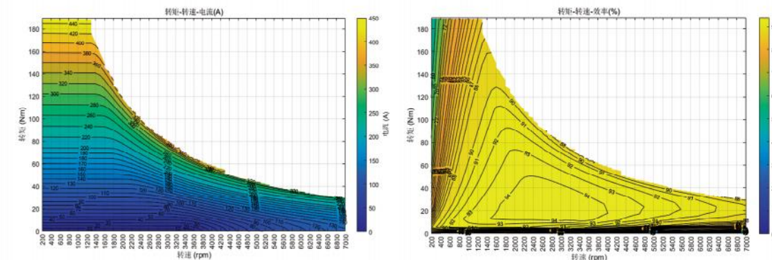
电流MAP
