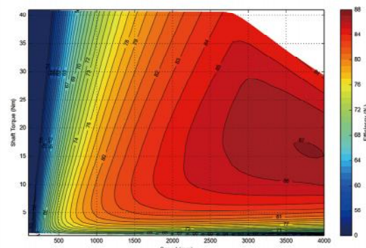
效率MAP
