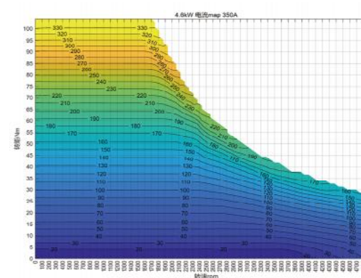
电流MAP
