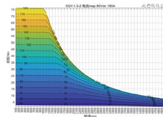
电流MAP
