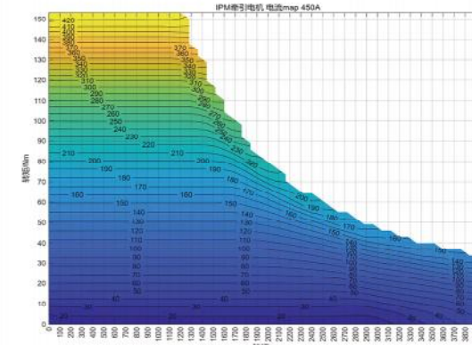
电流MAP
