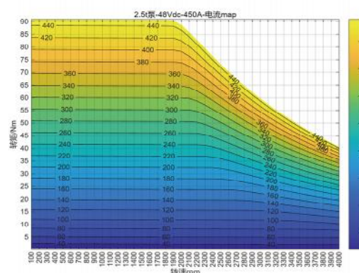
电流MAP
