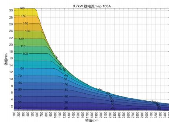
电流MAP
