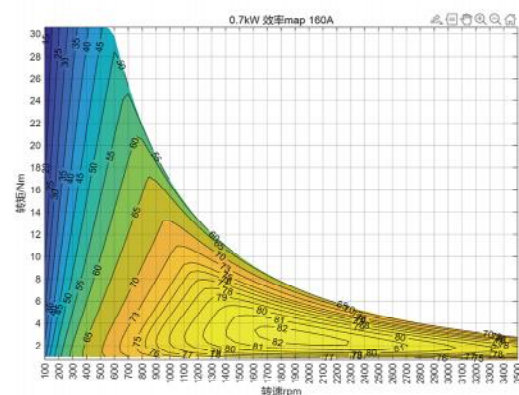
效率MAP
