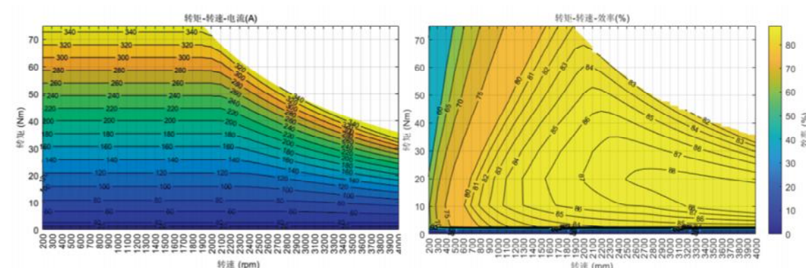
电流MAP
