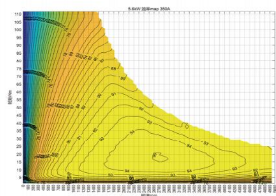
效率MAP
