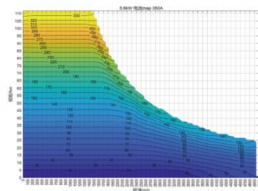
电流MAP
