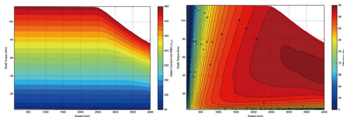
电流MAP
