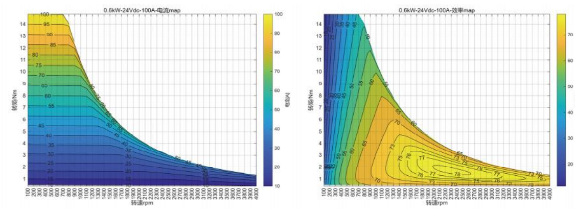
电流MAP
