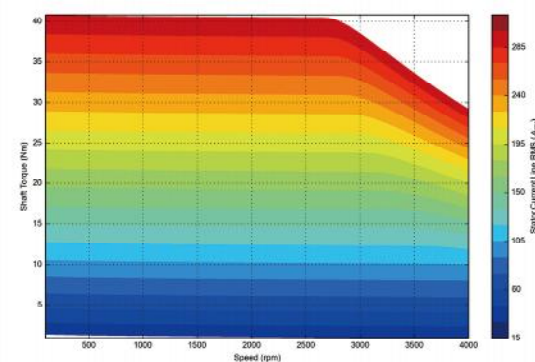
电流MAP
