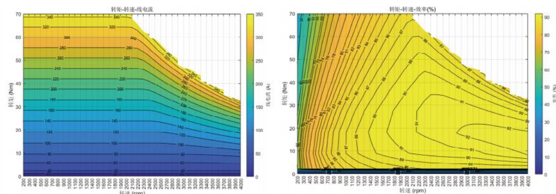
电流MAP
