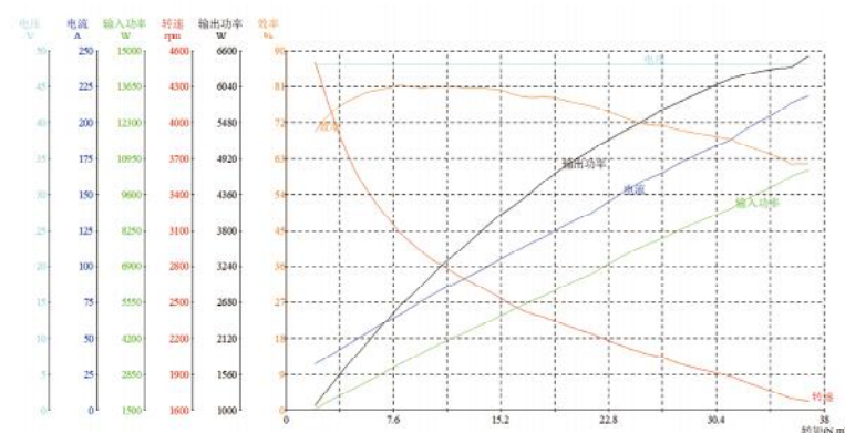
外特性
