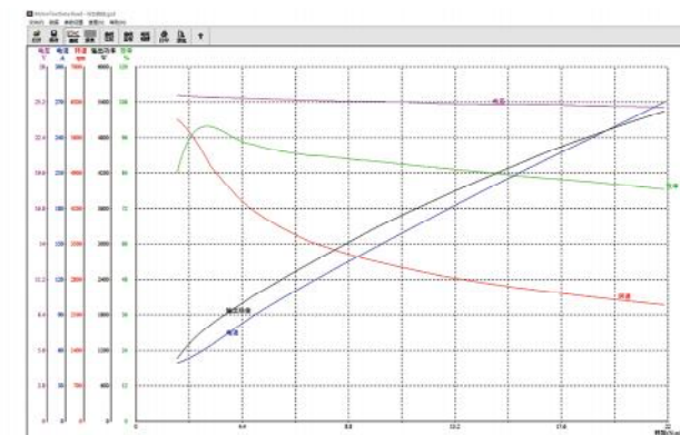
外特性
