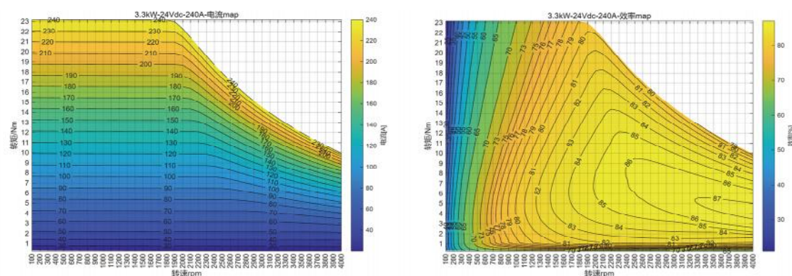
电流MAP
