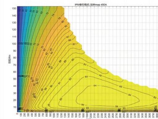
效率MAP
