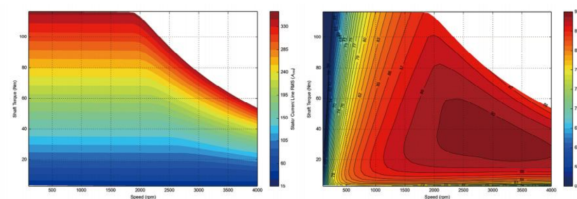
电流MAP
