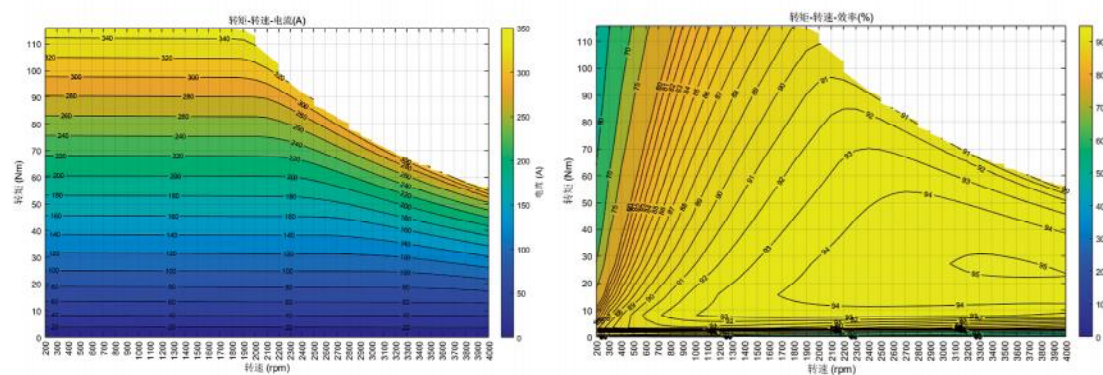
电流MAP
