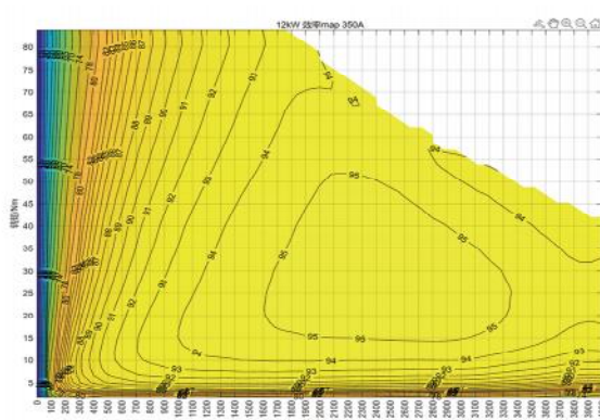
效率MAP
