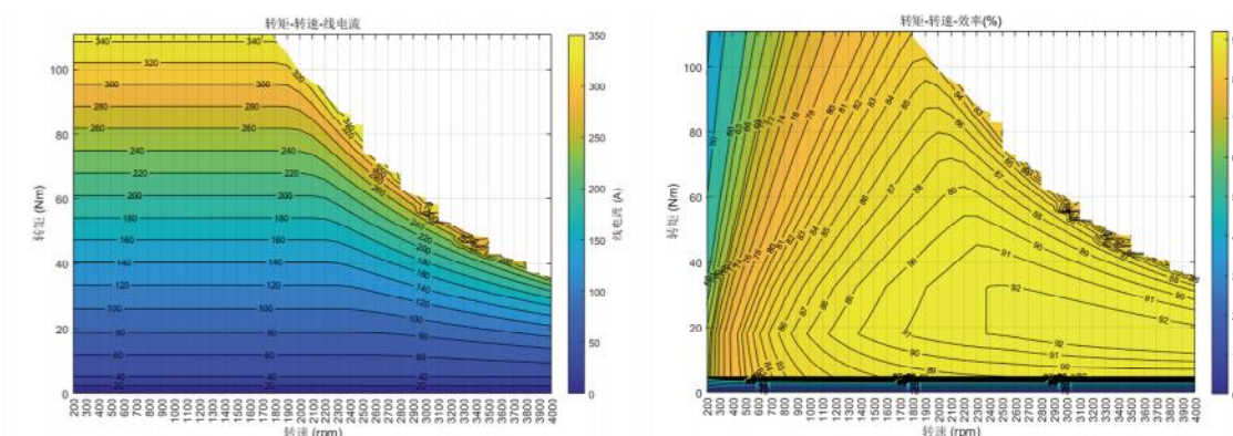
电流MAP
