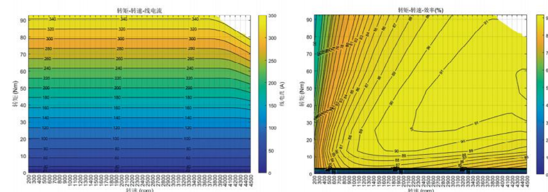
电流MAP
