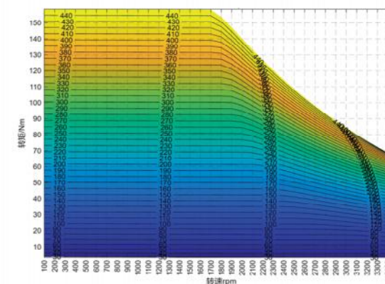
电流MAP
