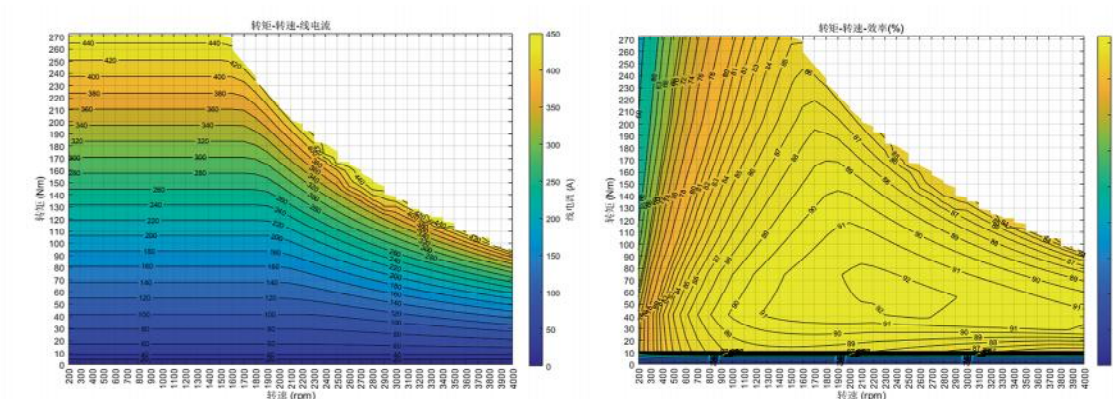
电流MAP
