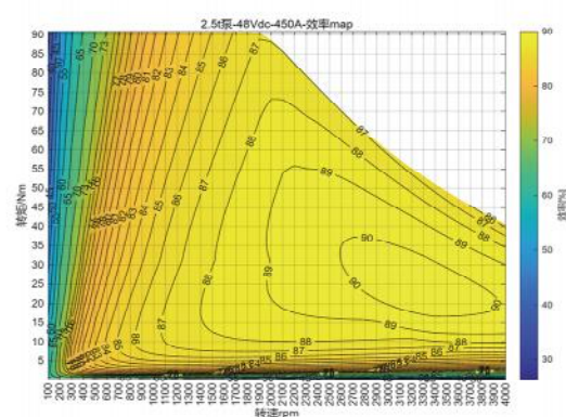
效率MAP
