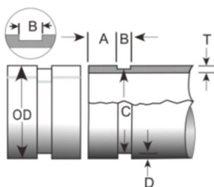
切槽短管
