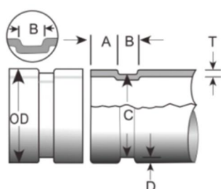
滚槽短管
