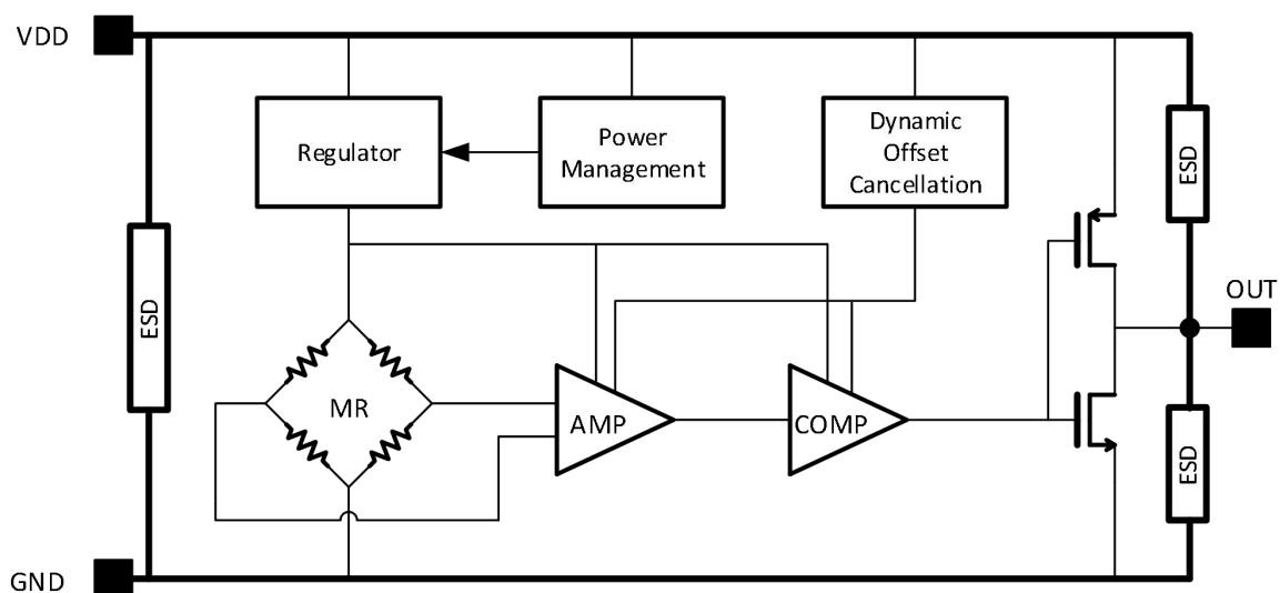
图 2 模块/线路图
